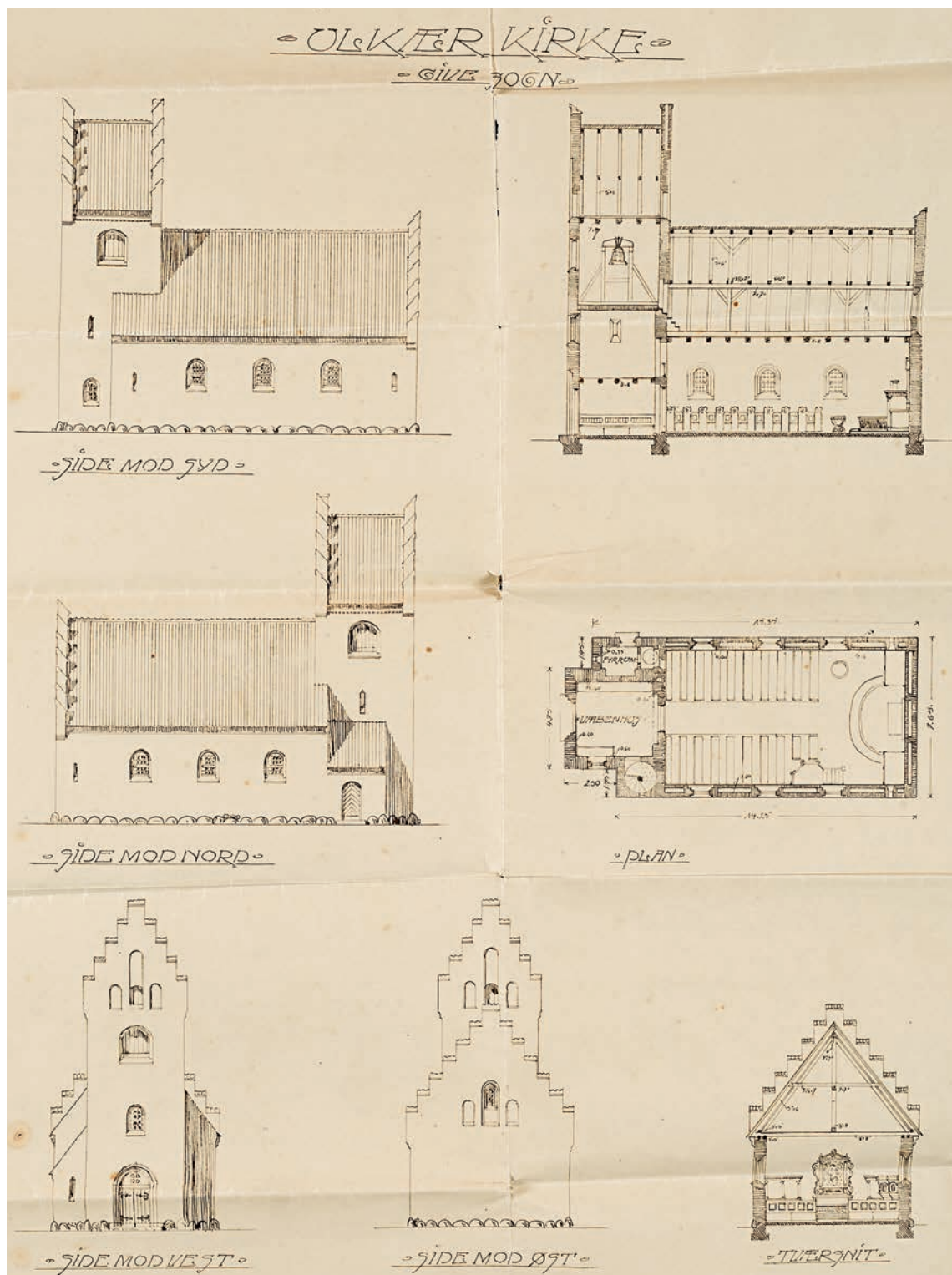
Fig. 8. Ikke anvendt projekt til mindre kirke i Ulkær (s. 2467). 1:300. Tegnet af Hother Paludan, 1919. Give-Egnens Museum og arkiv. — Unused proposal for a smaller church in Ulkær, 1919.
