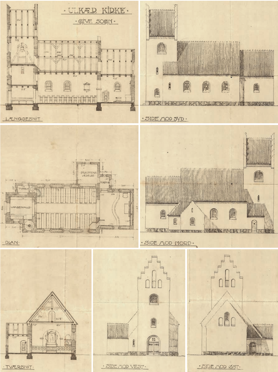
Fig. 7. Ikke anvendt projekt til kirke i Ulkær (s. 2467). 1:300. Tegnet af Hother Paludan, 1913. LAVib. – Unused proposal for a church in Ulkær, 1913.
