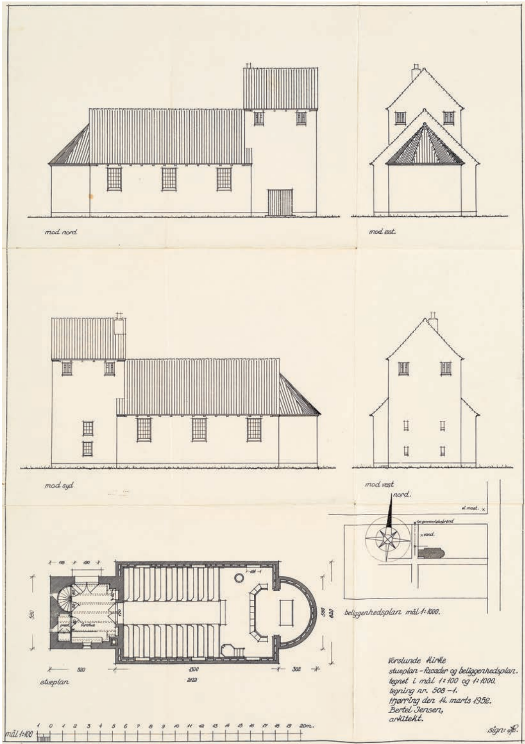
Fig. 3. Bertel Jensens bygningstegninger til kirken, 1952. 1:300. Give-Egnens Museum og arkiv. – Bertel Jensen's construction drawings for the church, 1952.
