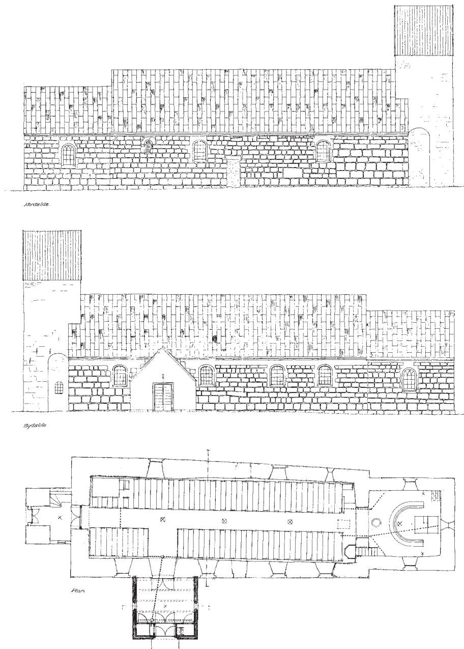
Fig. 6a-c. Opmåling af kirken. 1:300. a. Nordfacade. b. Sydfacade. c. Plan. Målt og tegnet af E. og F. M. R. Draiby 1951. — Scale drawings of the church. a. North facade. b. South facade. c. Ground plan.
