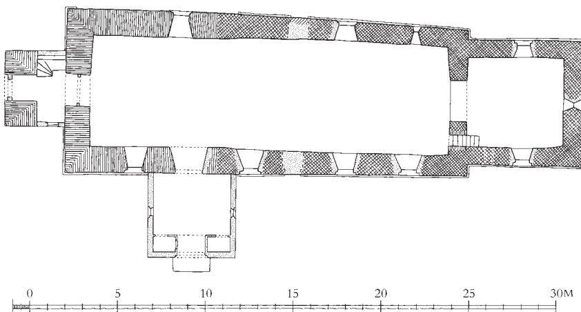
Fig. 5. Grundplan. 1:300. Målt af E. og F. M. R. Draiby 1951, suppleret af Niels Jørgen Poulsen og tegnet af Freerk Oldenburger 2017. Signaturforklaring s. 9. – Ground plan. Key on p. 17.
