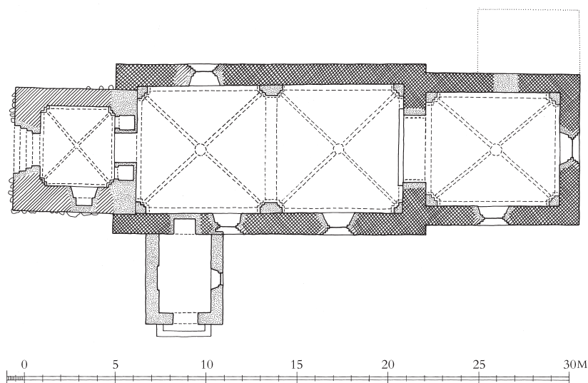
Fig. 5. Grundplan. 1:300. Målt af Kuno og Einar Mielby 2001, suppleret af Jakob Kieffer-Olsen og tegnet af Anders C. Christensen 2018. Signaturforklaring s. 9. – Ground plan. Key on p. 17.
