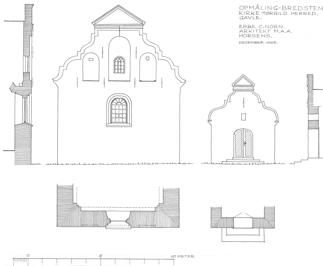
Fig. 50. Opstalter, planer og snit af korets og våbenhusets gavle (s. 2762). 1:150. Målt og tegnet af Ebbe C. Norn 1955. – Elevations, plans and sections of chancel and porch gables.
