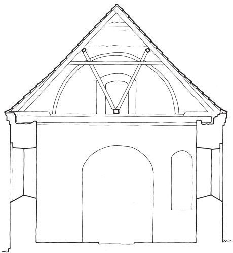
Fig. 8. Tværsnit gennem skib set mod øst. 1:150. Målt af Kuno Mielbye 1989, suppleret af Anders C. Christensen og Jakob Kieffer-Olsen, tegnet af Anders C. Christensen 2017. – Cross-section through nave looking east.
