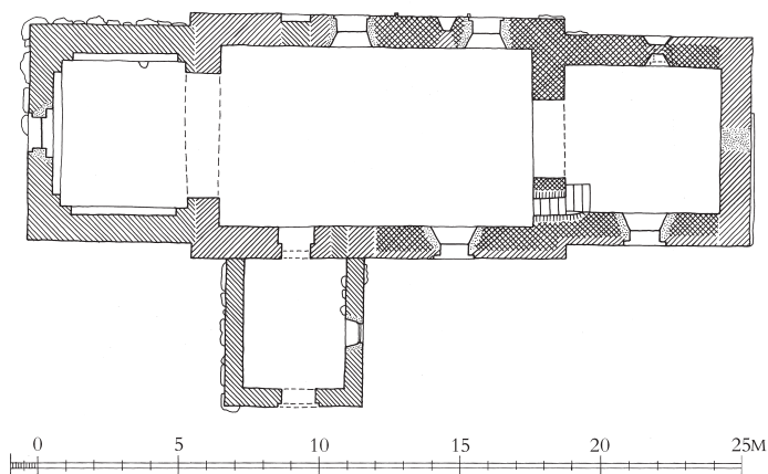
Fig. 5. Grundplan. 1:300. Målt af Kuno Mielbye 1989, suppleret af Jakob Kieffer-Olsen og tegnet af Anders C. Christensen 2017. Sig- naturforklaring s. 9. – Ground plan. Key on p. 17.
