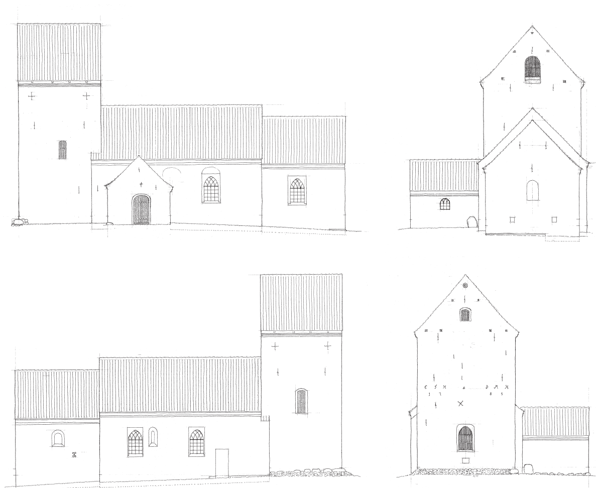
Fig. 10a–d. Opstalter af kirkens facader. 1:300. a. Sydfacade. b. Østfacade. c. Nordfacade (lisener ikke medtaget, jf. fig. 13 og 15). d. Vestfacade. Målt og tegnet af Kuno Mielbye 1989. – Elevations of the church facades. a. South facade. b. East facade. c. North facade. d. West facade.
