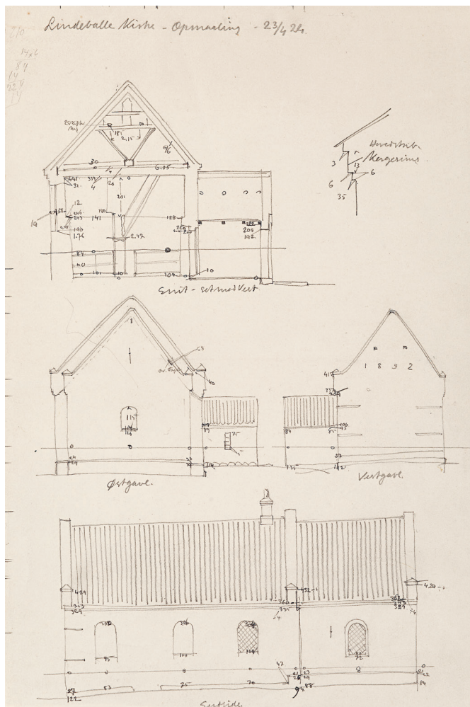
Fig. 37. Opmålingsskitse af kirken. C. Hess-Petersen, 1924. – Survey sketch of the church.
