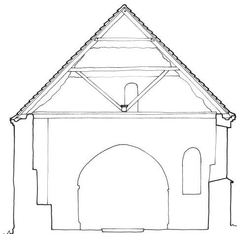
Fig. 10. Tværnsnit gennem skib set mod øst. 1:150. Målt af Anders C. Christensen og Jakob Kieffer-Olsen, tegnet af førstnævnte 2018. – Cross-section through nave seen towards the east.
