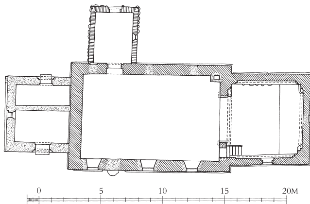
Fig. 9. Grundplan. 1:300. Målt af C. M. Smidt 1915 og C. Hess-Petersen 1924, suppleret af Jakob Kieffer-Olsen og tegnet af Anders C. Christensen 2019. Signaturforklaring s. 9. – Ground plan. Key on p. 17.
