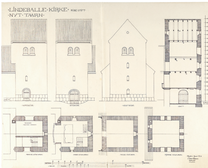
Fig. 14-15. Bygningstegninger af tårnet (s. 2861). C. Hess-Petersen 1924. — Construction drawings of the tower.
