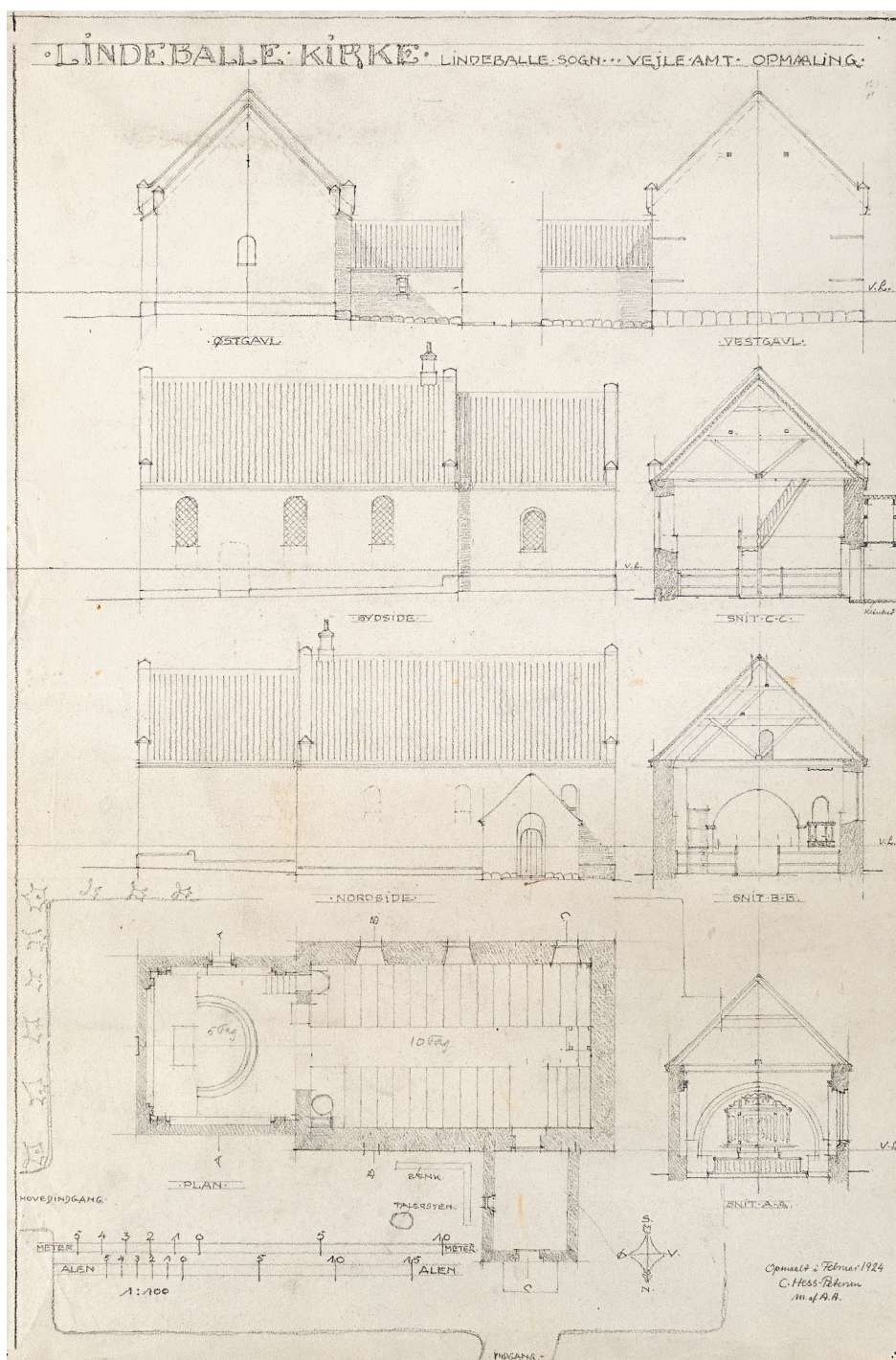
Fig. 13a-h. Opmåling af kirken. 1:300. a. Opstalt af østfacade. b. Opstalt af vestfacade. c. Opstalt af sydfacade. d. Tværnsnit af skib set mod vest. e. Opstalt af nordfacade. f. Tværnsnit af skib set mod øst. g. Plan. h. Tværnsnit af kor set mod øst. Målt af C. Hess-Petersen 1924. — Scale drawing of the church. a. Elevation of east facade. b. Elevation of west facade. c. Elevation of south facade. d. Cross-section of nave looking west. e. Elevation of north facade. f. Cross-section of nave looking east. g. Plan. h. Cross-section of chancel looking east.
