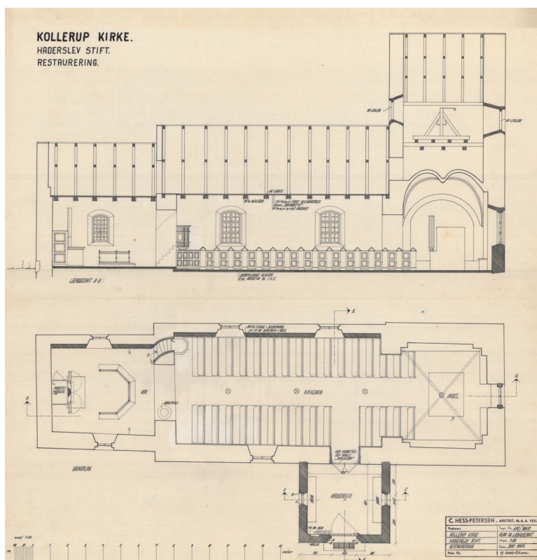
Fig. 15a. Restaureringsprojekt (s. 3220). 1:300. Længdesnit set mod syd og plan. Målt og tegnet af Carl Hess-Petersen 1949. – Restoration project by Carl Hess-Petersen 1949. Longitudinal section looking south and plan.
