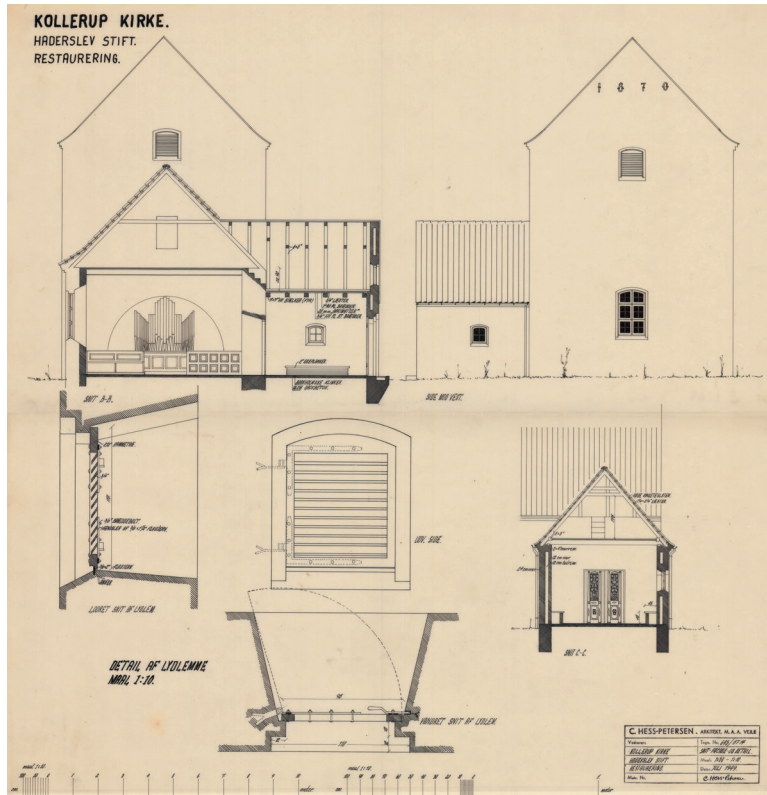
Fig. 15b. Restaureringsprojekt (s. 3220). 1:300. Tværsnit set mod vest, opstalt af vestfacade, tværsnit af våbenhus set mod syd samt detaljer. Målt og tegnet af Carl Hess-Petersen 1949. – Restoration project by Carl Hess-Petersen 1949. Cross-section looking west, elevation of west facade, cross-section of porch looking south and details.
