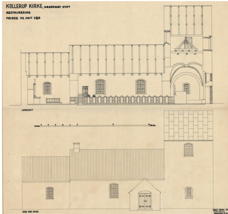
Fig. 67b. Restaureringsprojekt. 1:300. Længdesnit set mod syd og opstalt af nordfacade. Målt og tegnet af Carl Hess-Petersen 1944. – Restoration project by Carl Hess-Petersen, 1944. Longitudinal section looking south and elevation of north facade.
