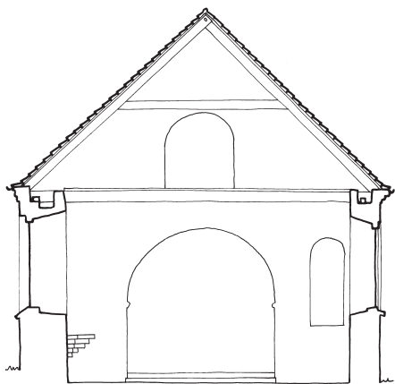
Fig. 5. Tværnit gennem skib set mod øst. 1:150. Målt af Anders C. Christensen og Jakob Kieffer-Olsen, tegnet af Anders C. Christensen 2021. – Cross-section through the nave, looking east.
