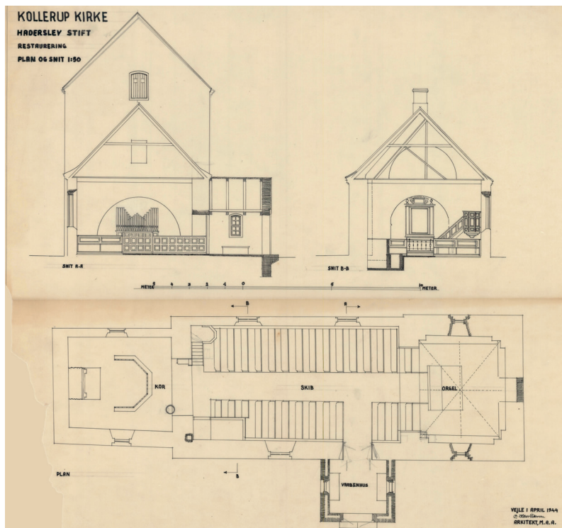
Fig. 67a. Restaureringsprojekt. 1:300. Tværnsnit set mod vest og øst samt plan. Målt og tegnet af Carl Hess-Petersen 1944. – Restoration project by Carl Hess-Petersen, 1944. Cross-sections of nave looking west and east and plan.
