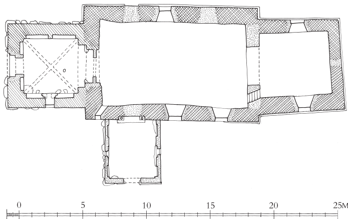
Fig. 6. Plan. 1:300. Målt af Kristian Pedersen 1976, suppleret og tegnet af Anders C. Christensen 2022. Signaturforklaring s. 9. – Plan. Key on p. 17.
