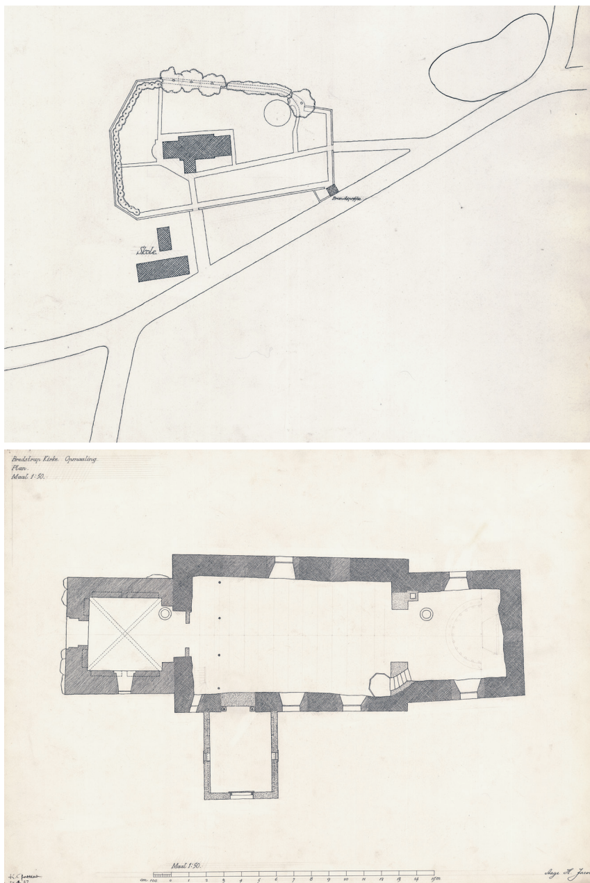
Fig. 21a-b. Opmålinger. a. Situationsplan. 1:2000. b. Plan. 1:300. Målt og tegnet af Aage H. Jacobsen 1936-37. I Danmarks Kunstbibliotek. — Scale drawings. a. Location plan. b. Plan.
