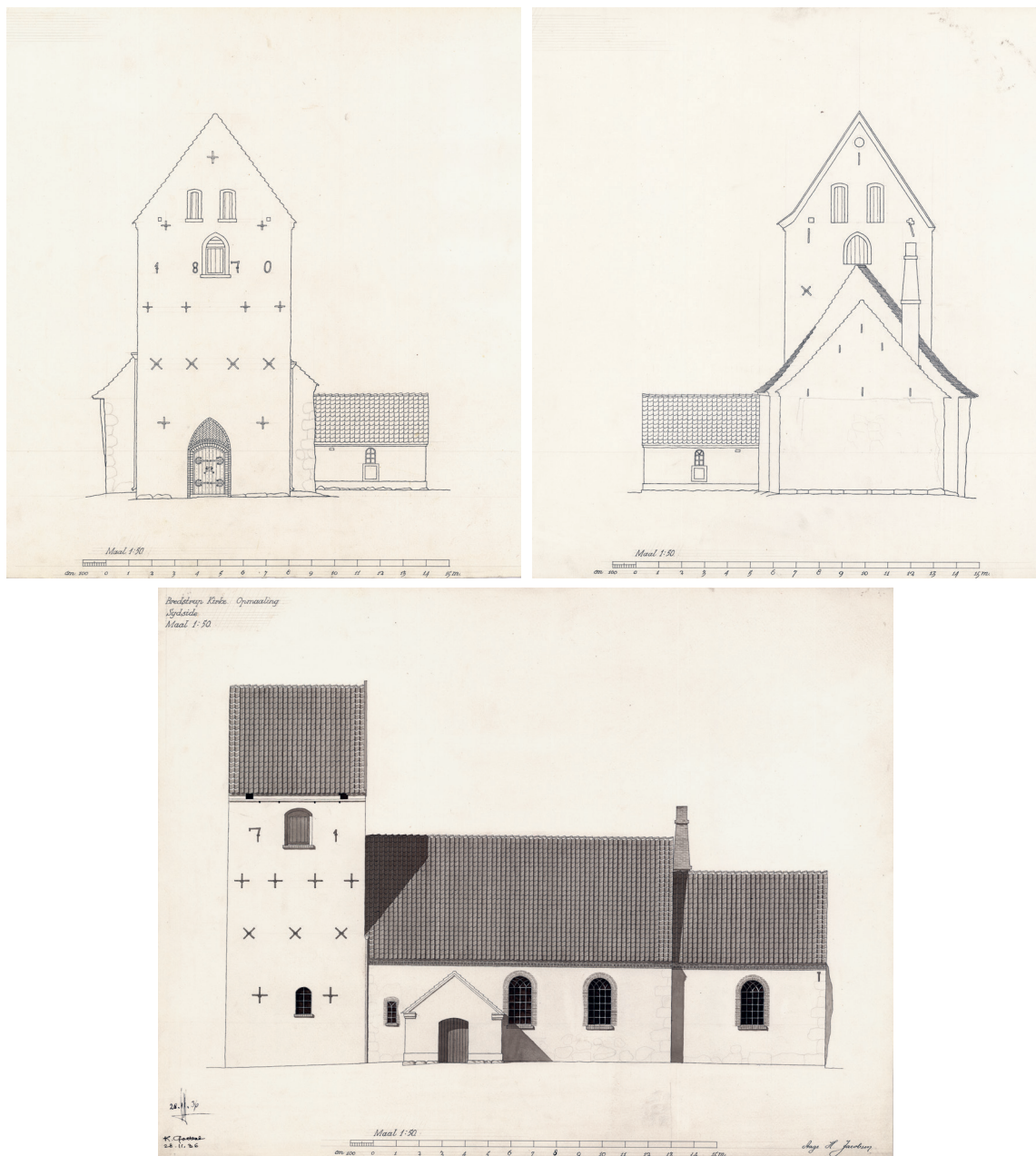
Fig. 21c-e. Opmålinger. 1:300. c. Opstalt af vestfacade. d. Opstalt af østfacade. e. Opstalt af sydfacade. Målt og tegnet af Aage H. Jacobsen 1936-37. I Danmarks Kunstbibliotek. – Scale drawings. c. Elevation of west facade. d. Elevation of east facade. e. Elevation of south facade.
