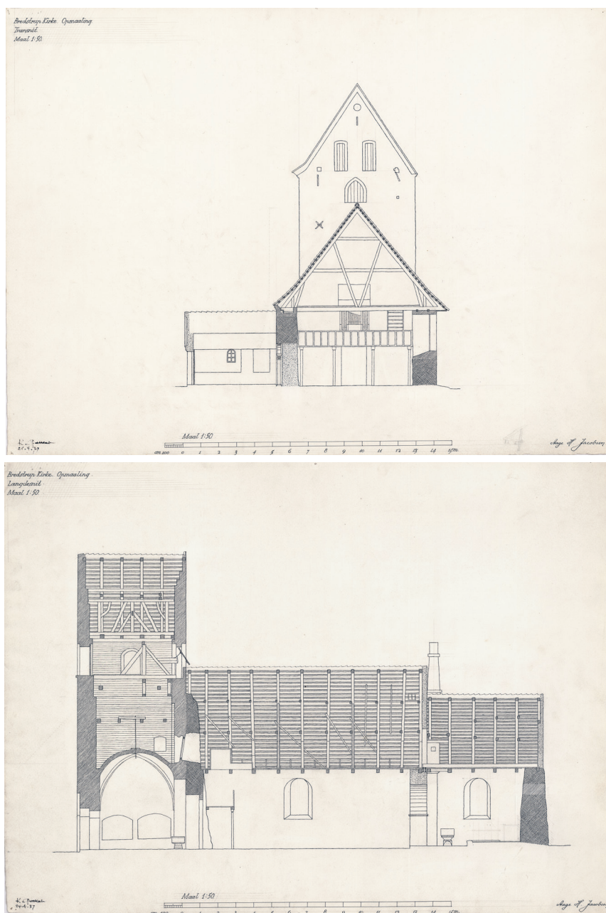
Fig. 21f-g. Opmålinger. 1:300. f. Tværsnit af skib set mod vest. g. Længdesnit set mod nord. Målt og tegnet af Aage H. Jacobsen 1936-37. I Danmarks Kunstmuseum. — Scale drawings. f. Cross-section looking west. g. Longitudinal section looking north.
