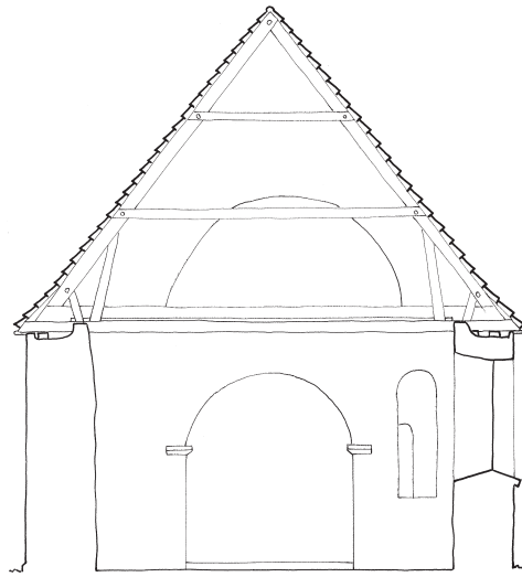
Fig. 7. Tværsnit gennem skibet set mod øst. 1:150. Målt og tegnet af Anders C. Christensen 2022. – Cross section through the nave seen from the east.
