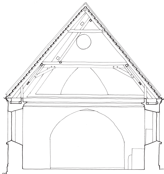
Fig. 6. Tværsnit gennem skibet set mod øst. 1:150. Målt og tegnet af Anders C. Christensen 2022. – Cross section through the nave looking east.
