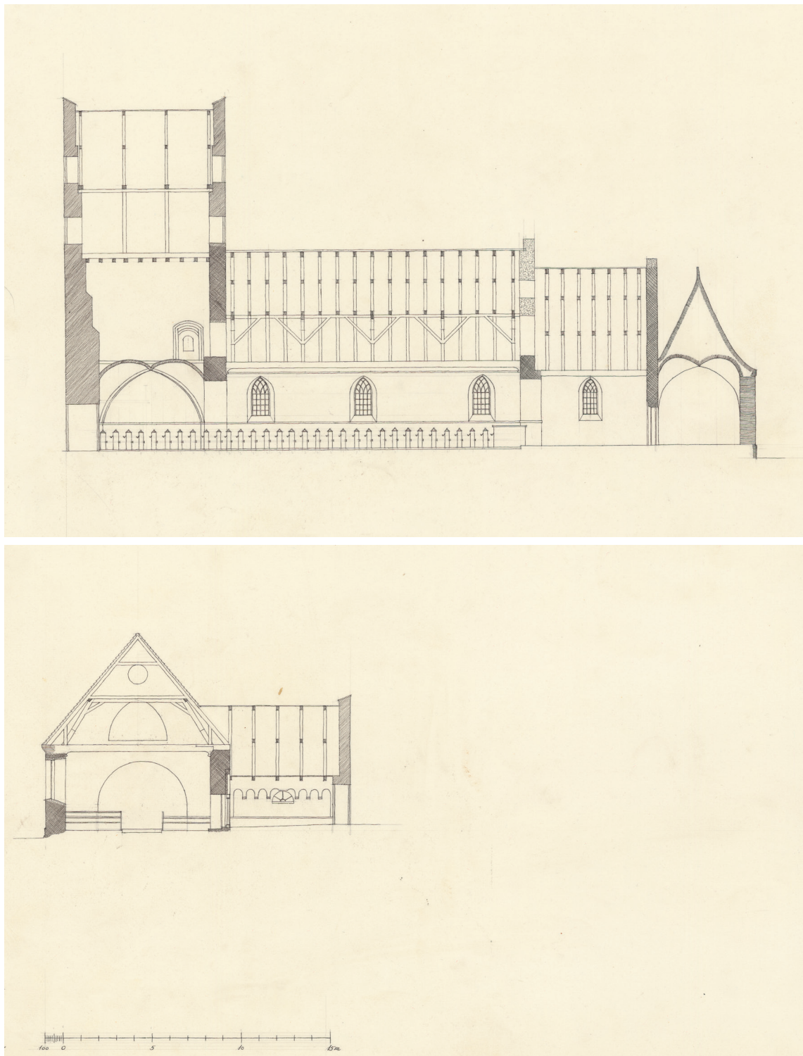
Fig. 27f-g. Opmålinger. 1:300. f. Længdesnit set mod nord. g. Tværsnit af skib set mod øst. Målt og tegnet af Ove R. Nielsen 1934. I Danmarks Kunstbibliotek. — Scale drawings. f. Longitudinal section looking north. g. Cross-section looking east.
