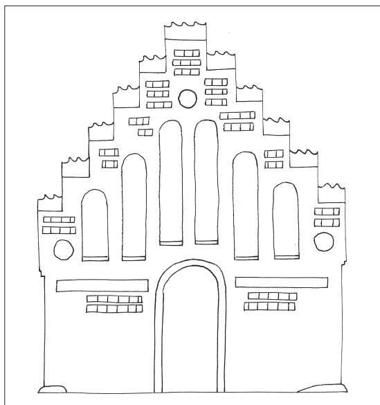
Fig. 70. Opstalt af våbenhusets sydgavl (s. 3741). 1:100. Målt og tegnet af Anders C. Christensen 2021. – Elevation of the south gable of the porch.
