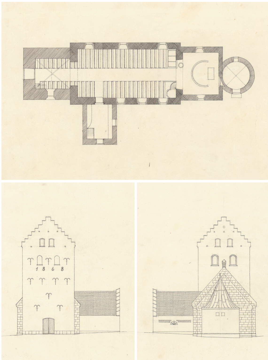
Fig. 27a-c. Opmålinger. 1:300. a. Plan. b. Opstalt af vestfacade. c. Opstalt af østfacade. Målt og tegnet af Ove R. Nielsen 1934. I Danmarks Kunstbibliotek. — Scale drawings. a. Plan. b. Elevation of west facade. c. Elevation of east facade.
