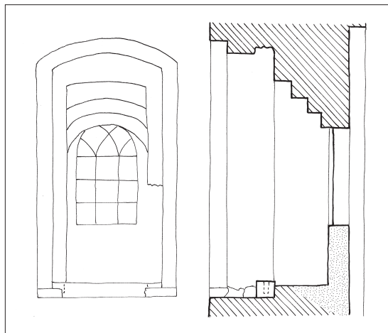
Fig. 71. †Dør i tårnets mellemstokværk (s. 3744). Opstalt af inderside og snit set mod vest. 1:50. Målt og tegnet af Anders C. Christensen 2022. – Door in the middle storey of the tower. Elevation of inside and section.
