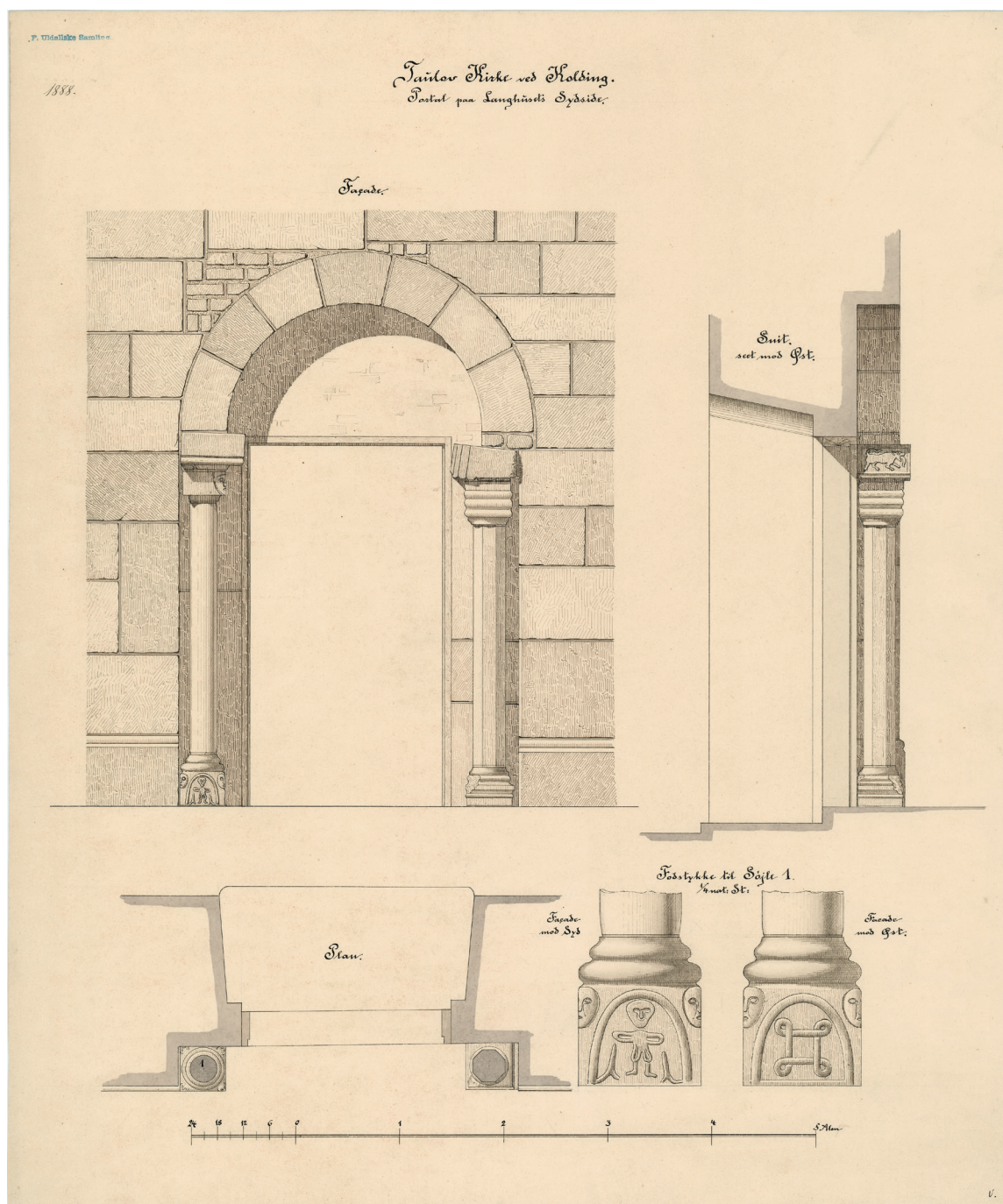
Fig. 8. Skibets sydportal (s. 3734). 1:40. Opmåling ved F. Uldall 1888. I NM. — South portal of the nave.
