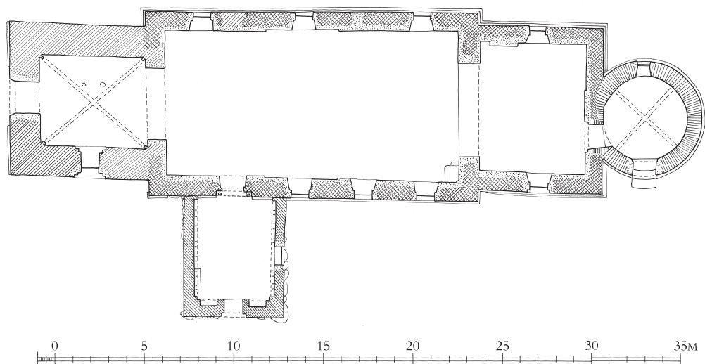
Fig. 7. Plan. 1:300. Målt af Ebbe Lehn Petersen 1958, suppleret og tegnet af Anders C. Christensen 2022. Signaturforklaring s. 9. – Plan. Key on p. 17.
