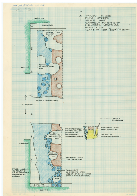
Fig. 72. Ældre fundament i skibets vestende (s. 3733). 1:100. Målt og tegnet af Birgit Als Hansen 1981. I NM. – Old foundations in the west end of the nave.
