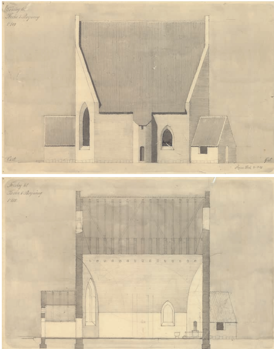
Fig. 6a-c. Tegninger. 1:300. a. (tv.) Plan. b. Opstalt af sydfacade. c. Længdesnit set mod nord. Skitser ved Mogens Koch 1941. Mogens Koch Design I/S. – Drawings. a. (left) Plan. b. Elevation of south facade. c. Longitudinal section looking north.
