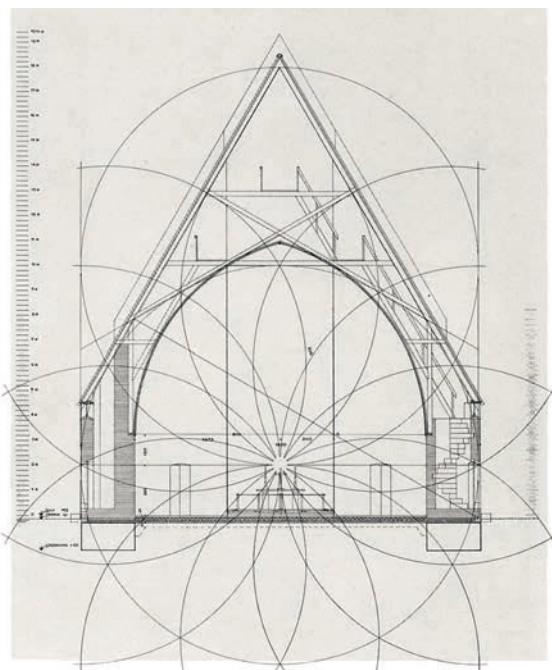
Fig. 21a. Geometriske principper, tværsnit. 1:300. Efter Karlsen 1968. – Geometric principles, cross section .
