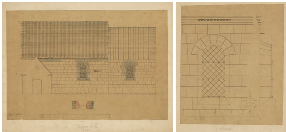
Fig. 19a-b. Sydfacade samt detalje af nye vinduer (s. 3903). 1:300 og 1:75. Målt og tegnet Mogens L. Hansen. – South facade and detail of new windows.
