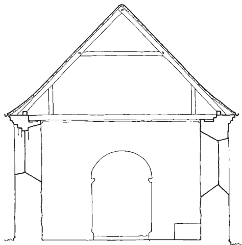
Fig. 8. Tværsnit gennem skibet set mod øst. 1:150. Målt og tegnet af Anders C. Christensen 2023. – Cross section through the nave facing east.
