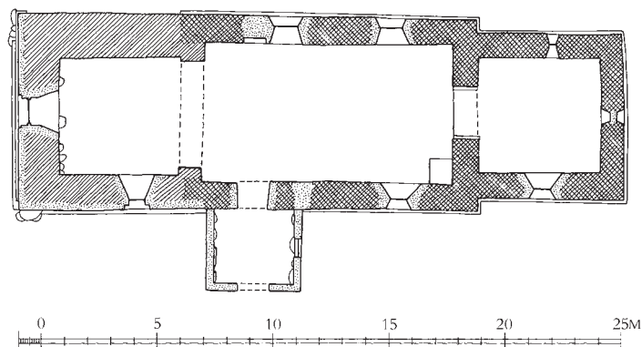
Fig. 7. Plan. 1:300. Målt af Aksel Skov 1959, suppleret og tegnet af Anders C. Christensen 2023. Signaturforklaring s. 9. – Plan. Key on p. 17.
