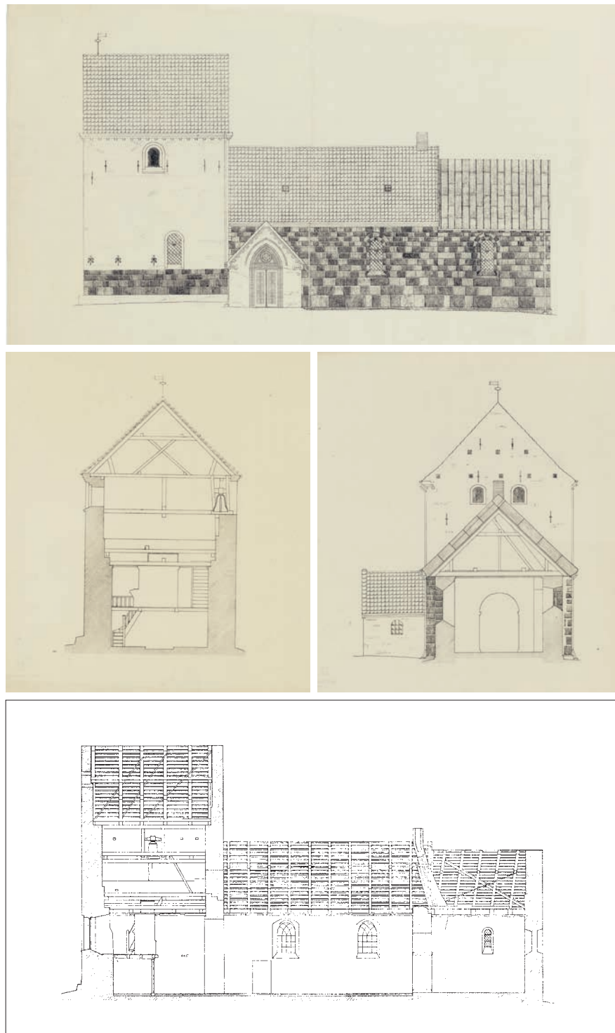
Fig. 17a-d. Opmålinger. 1:300. O. 1962. a. Sydfacade. b. Tværnsnit gennem tårn set mod vest. c. Tværnsnit gennem kor set mod vest. d. Længdesnit set mod nord. — Scale drawings. a. South facade. b. Cross-section of tower looking west. c. Cross section of chancel looking west. d. Longitudinal section looking north.
