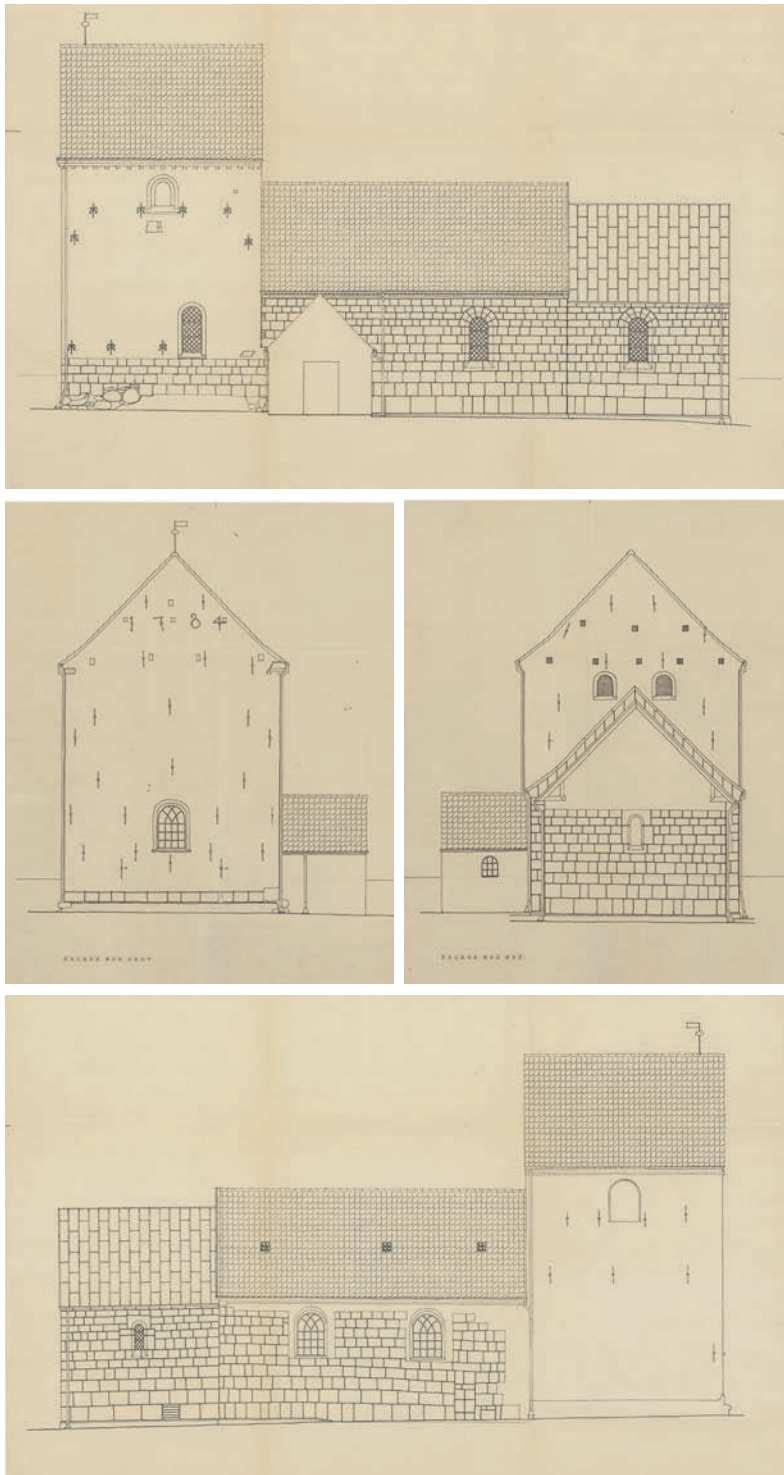
Fig. 18a-d. Opmålinger. 1:300. Målt og tegnet af Kuno Mielby 1986-88. a. Sydfacade. b. Vestfacade. c. Østfacade. d. Nordfacade. — Scale drawings. a. South facade. b. West facade. c. East facade. d. North facade.
