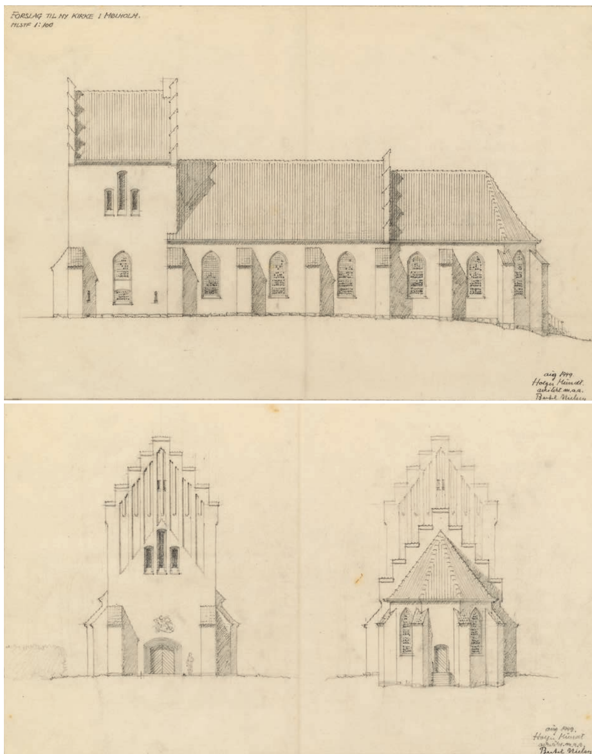
Fig. 25a-b. Forslag til kirke. 1:300. Tegnet af Holger Mundt og Bertel Nielsen 1949. I Danmarks Kunsthbibliotek. a. Sydfacade. b. Vest- og østfacade. – Proposal for church. a. South facade. b. West and east facade.
