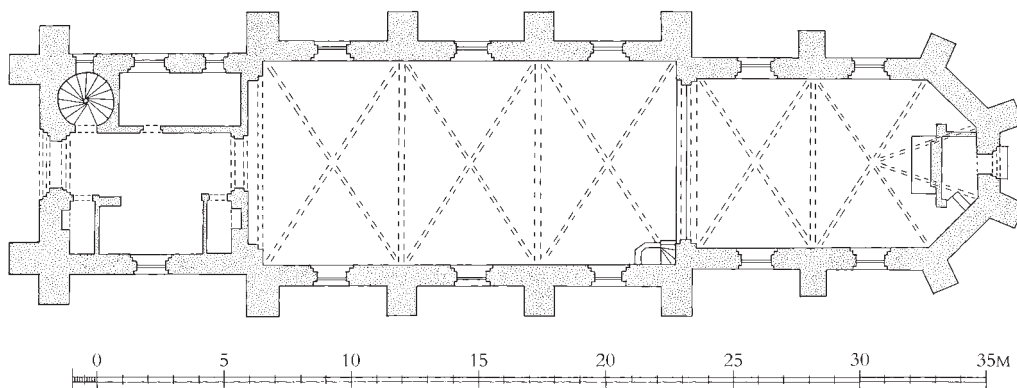
Fig. 6. Plan. 1:300. Holger Mundt og Bertel Nielsen 1950, suppleret af Anders C. Christensen og tegnet af Freerk Oldenburger 2023. Signaturforklaring s. 9. – Plan. Key on p. 17.
