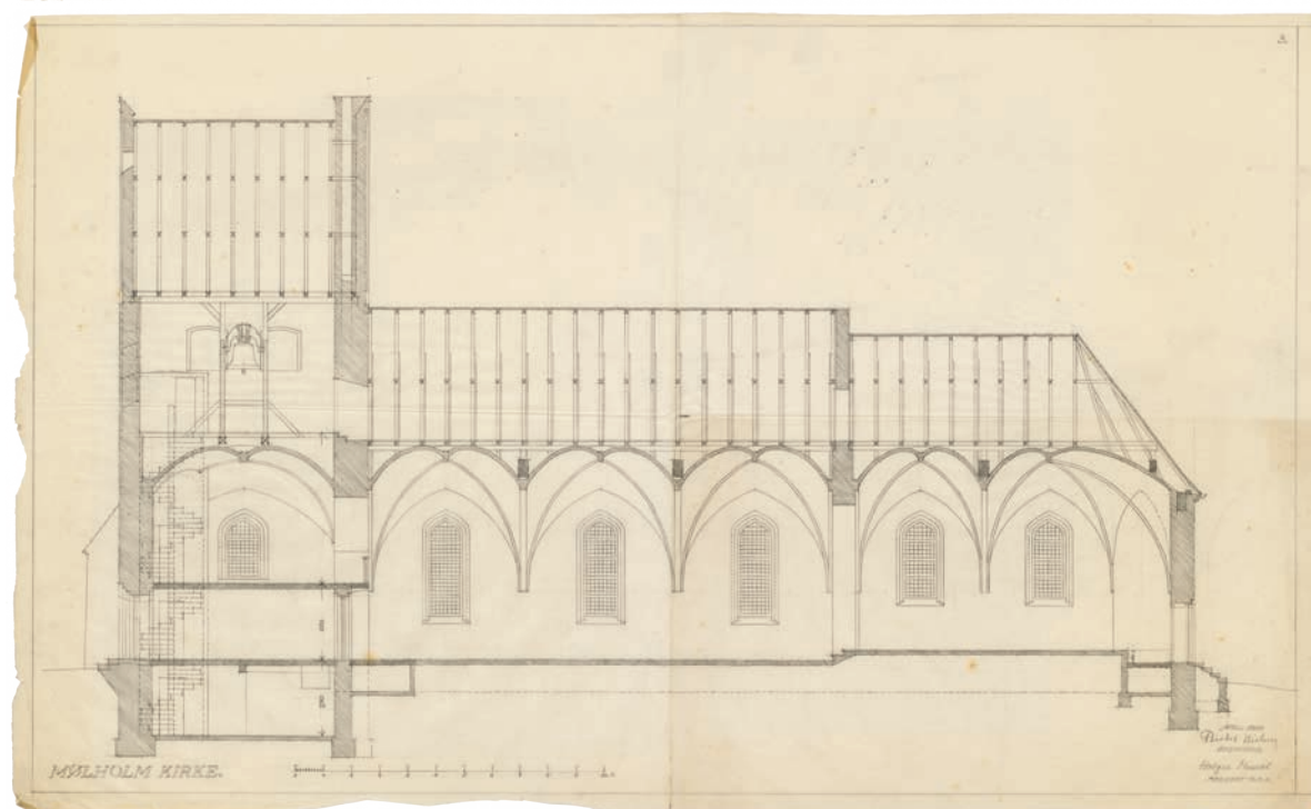
Fig. 7a-b. Projekt til kirke. 1:300. Tegnet af Holger Mundt og Bertel Nielsen 1950. I Danmarks Kunsthbibliotek. a. Sydfacade. b. Længdesnit set mod nord. – Layout of church. a. South facade. b. Longitudinal section looking north.
