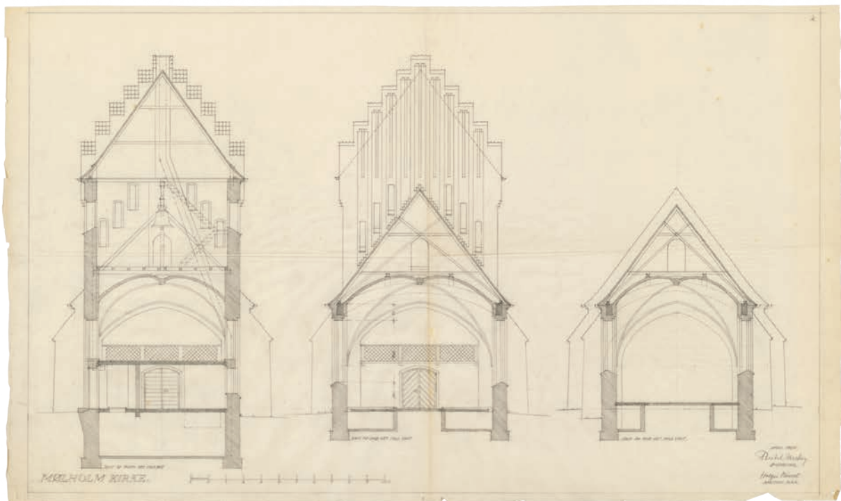
Fig. 7c-d. Projekt til kirke. 1:300. Tegnet af Holger Mundt og Bertel Nielsen 1950. I Danmarks Kunstbibliotek. c. Plan. d. Tværsnit af tårn set mod øst, tværsnit af skib set mod vest og tværsnit af kor set mod vest. — Layout of church. c. Plan. d. Cross section of tower looking east, cross section of nave looking west and cross section of chancel looking west.
