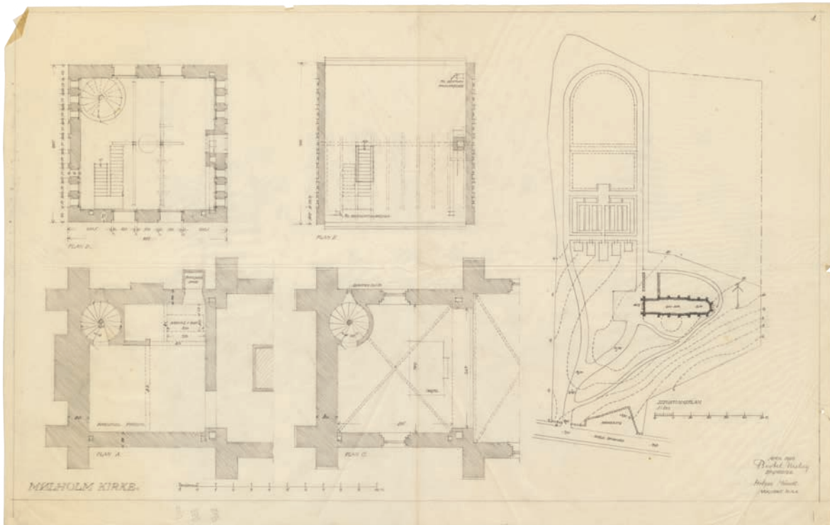
Fig. 26. Projekt til kirke (jf. fig. 7a-d). 1:300 og 1:3000. Planer af tårnets fyrcælder, pulpiturstokværk, klokkestokværk og loftsrum samt situationsplan. Tegnet af Holger Mundt og Bertel Nielsen 1950. I Danmarks Kunstbibliotek. – Layout of church (see fig. 7a-d). Plans of the tower's boiler room, gallery floor, belfry and loft, as well as location plan.
