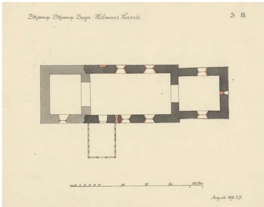
Fig. 19a-b. Opmålinger. Målt og tegnet af Erik Schiødte 1878. I NM. a. Korets østvindue og skibets syddør. 1:50. b. Plan. 1:300. — a. The east window of the chancel and the south door of the nave. b. Plan.
