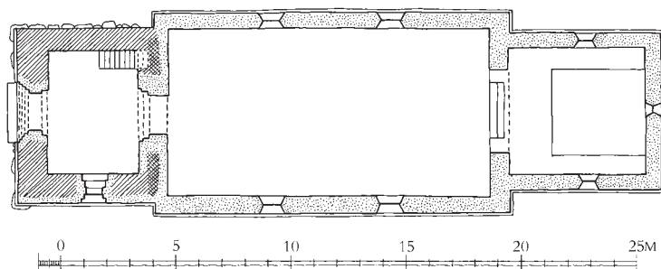
Fig. 6. Plan. 1:300. Signaturforklaring s. 9. Målt og tegnet af Anders C. Christensen 2023. – Plan. Key on p. 17.
