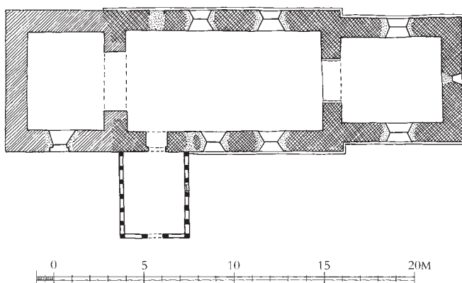
Fig. 18. Plan af nedrevne kirke. 1:300. Erik Schiødte 1878, suppleret og tegnet af Anders C. Christensen 2023. Signaturforklaring s. 9. – Plan of demolished church. Key on p. 17.
