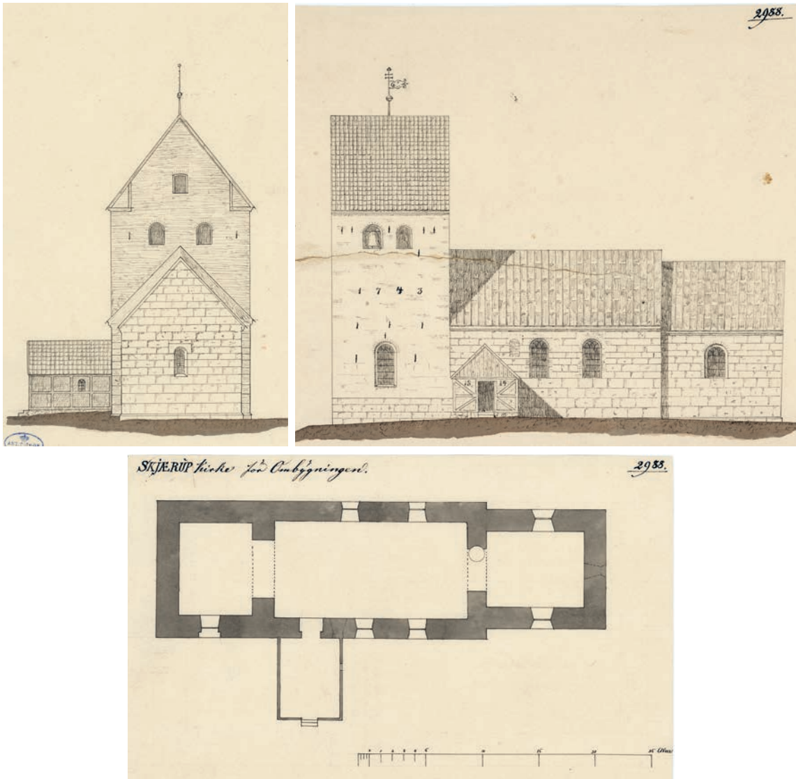
Fig. 21a-c. Tegninger. 1:300. a-b. Opstalter af øst- og sydfacader. c. Plan. L. A. Winstrup o. 1880. I NM. – a-b. Elevations of east and south sides. c. Plan
