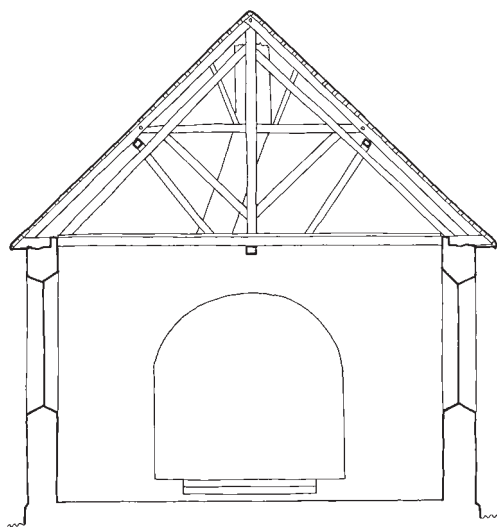
Fig. 5. Tværsnit gennem skibet set mod øst. 1:150. Målt og tegnet af Anders C. Christensen 2023. – Cross section through the nave looking east.
