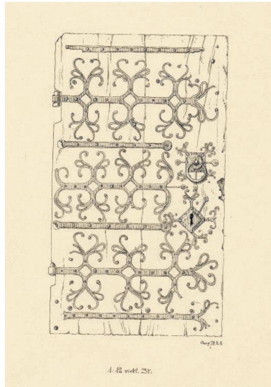
Fig. 86c. Den senmiddelalderlige dørføj (s. 4140). 1:50. Målt og tegnet af Erik Schiødt 1878. I NM. – The Late Medieval door wing .
