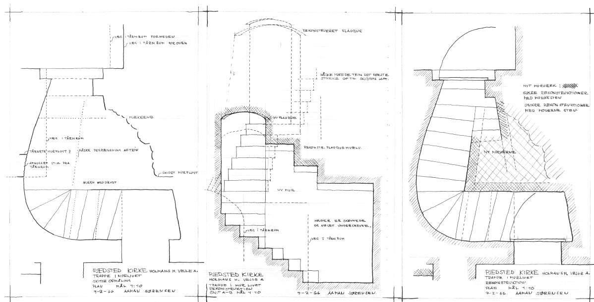
Fig. 27a-c. a. Skitseopmåling af tårnopgang, plan (s. 4106). b-c. Rekonstruktionstegning af trappeopgang, snit set mod syd og plan (s. 4114). 1:50. Målt og tegnet af Morten Aamann Sørensen 1966. I NM. – a. Scale drawing of tower stairway, plan. b-c. Reconstruction drawing of stairway, section looking south, and plan.
