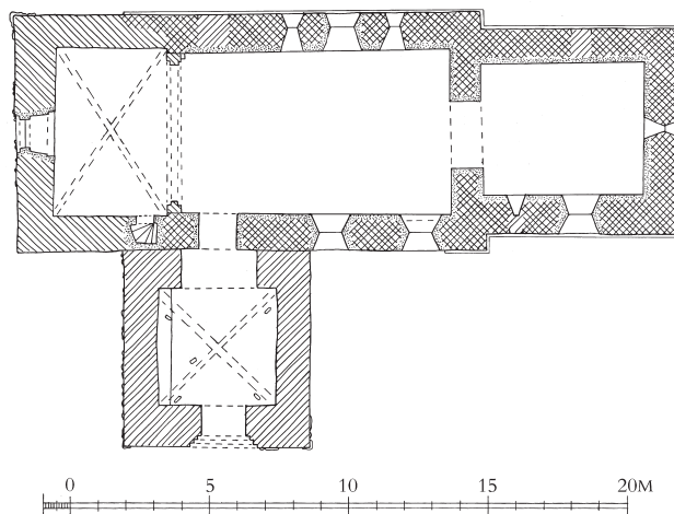
Fig. 15. Plan. 1:300. Målt og tegnet af Line M. Bonde 2024. Signaturforklaring s. 9. – Plan. Key on p. 17.
