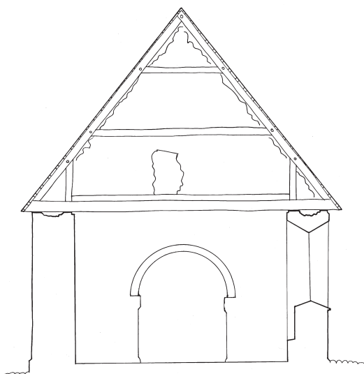
Fig. 13. Tværsnit gennem skibet set mod øst. 1:150. Målt og tegnet af Line M. Bonde 2024. – Cross-section through the nave looking east.
