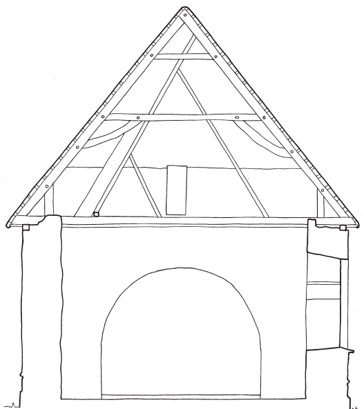
Fig. 8. Tværsnit gennem skibet set mod øst. 1:150. Målt og tegnet af Anders C. Christensen 2023. – Cross section of the nave looking east.
