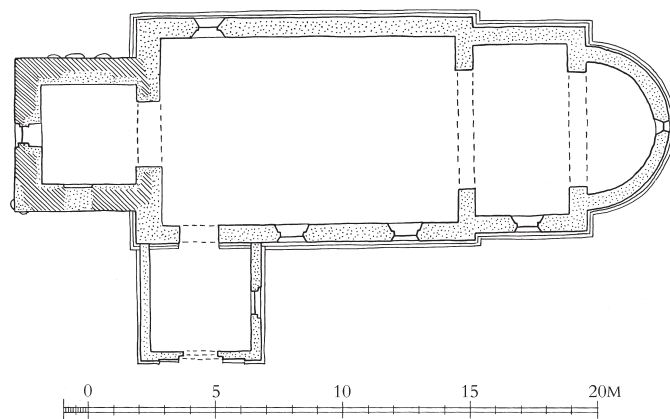
Fig. 5. Plan. 1:300. Målt af S.A.Aakjær og H. Lund 1987, suppleret og tegnet af Anders C. Christensen 2024. Signaturforklaring s. 9. – Plan. Key on p. 17.
