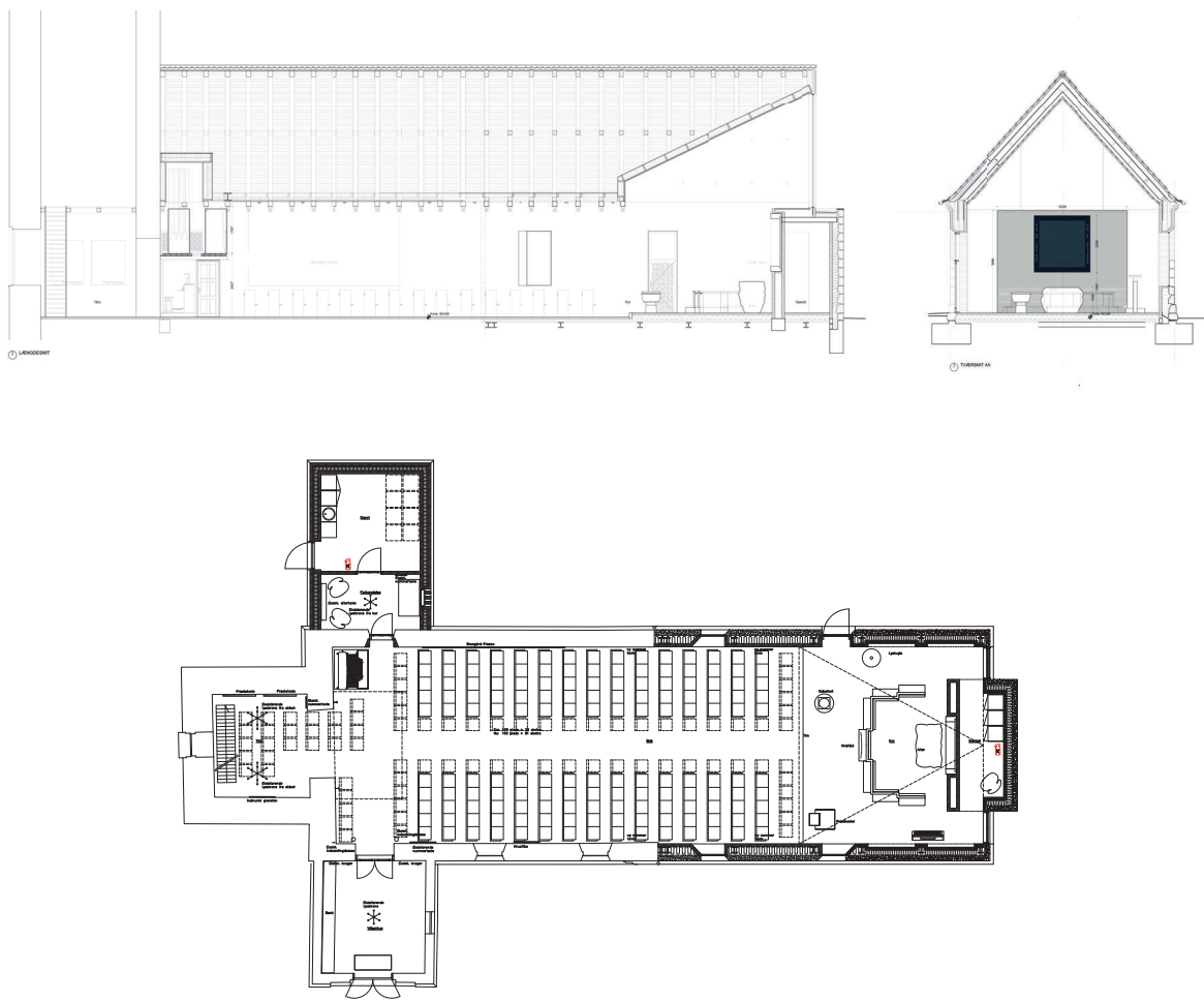
Fig. 14a-c. Længde- og tværsnit samt plan af udvidet kirke. 1:300. R Arkitekter 2024. – Longitudinal and cross section and plan of extended church.
