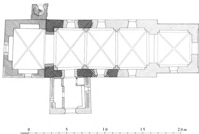
Fig. 2. Plan. 1:300. Målt af MB 1959. Tegnet af HJ 1980. Signaturforklaring s. 9.
