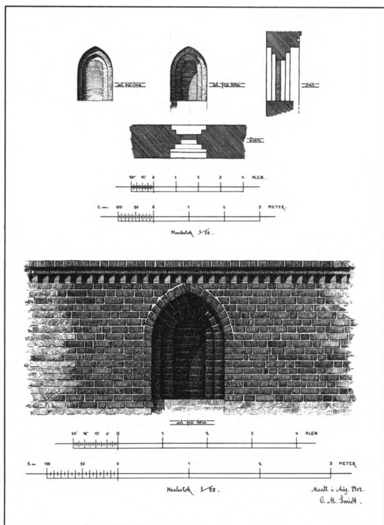
Fig. 8. Langhuskorets nordvindue (s. 1303). Plan, opstalt og snit samt udvendig facade, nu mod sakristiets loft. 1:150 og 1:75. Målt og tegnet af
