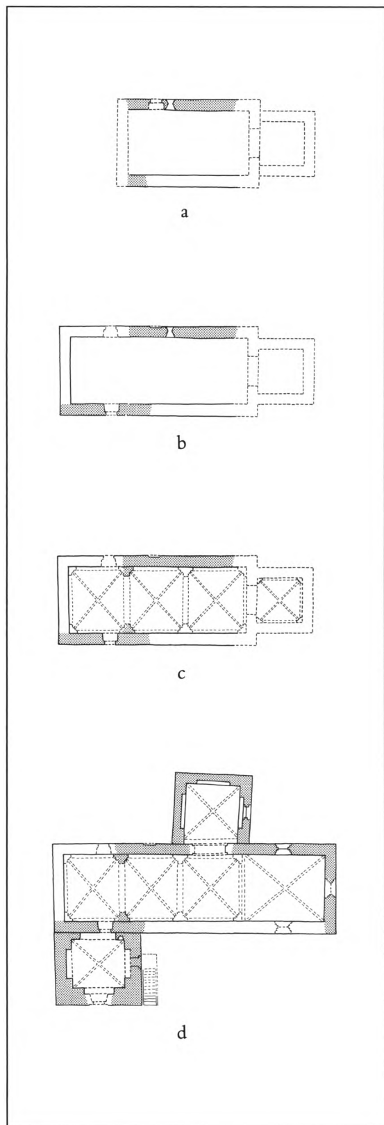
Fig. 4. Hovedetaper i kirkens middelalderlige bygningshistorie. Skematiske planer med angivelse af bevaret murværk samt sikre og formodede murforløb. 1:400. Rekonstruktion ved HJ, tegnet af Marianne Nielsen 1985. a. Senromansk kirke o. 1200 (s. 1299). b. Vestforlængelse af skibet o. 1250-1350 (s. 1300). c. Hvælvslægning i den forlængede kirke (s. 1301). d. Omdannelse til langhus med kor fra o. 1375-1400 (s. 1301), hvortil i 1400'rne er føjet tårn med våbenhus i underetagen (s. 1303) samt et kapel mod nord (s. 1305). e. Opførelse af sideskib ved kirkens sydside o. 1500. Planlagte hvælv er angivet (s. 1307). f. Hvælvslægning i søndre sideskib (s. 1308). g. Omdannelse til toskibet hallekirke o. 1525 (s. 1308) med lidt yngre sakristi i nord (s. 1310). Endvidere er angivet omdannelsen af nordkapellet til våbenhus som følge af indretning af lukket gravkapel i tårnet i 1600'rne (s. 1307). - Principal phases of the church's medieval building history. Schematic plans showing preserved wall, as well as unquestionable and supposed courses of wall. 1:400. a. Late Romanesque church c. 1200. b. West extension of the nave c. 1250-1350. c. Vaulting in the extended church. d. Rebuilt as long-house with chancel c. 1375-1400; a tower with porch in the first storey was added in the 1400s, and a chapel to the north. e. Side aisle built on to the south wall. c. 1500, proposed vaults are shown. f. Vaults in the south side aisle. g. Rebuilt as a hall church with two aisles c. 1525, and with a slightly later sacristy to the north. Also shown is the rebuilt north chapel now the porch after the ground-floor tower chamber had been turned into a closed burial vault in the 1600s.
