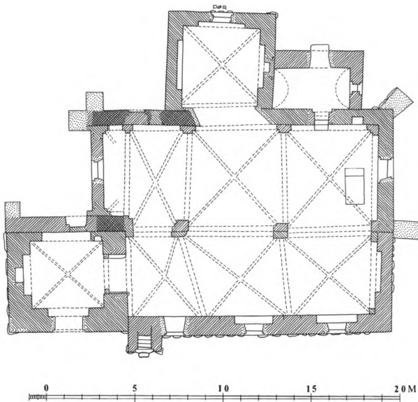
Fig. 3. Plan. 1:300. Målt af MB 1966, tegnet af Marianne Nielsen 1985. Signaturforklaring s. 9. - Ground-plan Key on p. 9.
