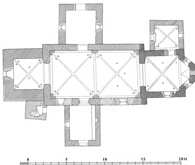
Fig. 2. Plan. 1:300. Målt af Charles Christensen 1921, revideret af HJ 1985 og tegnet af Marianne Nielsen 1986. Signaturforklaring s. 9. - Ground-plan. Key on p. 9.
