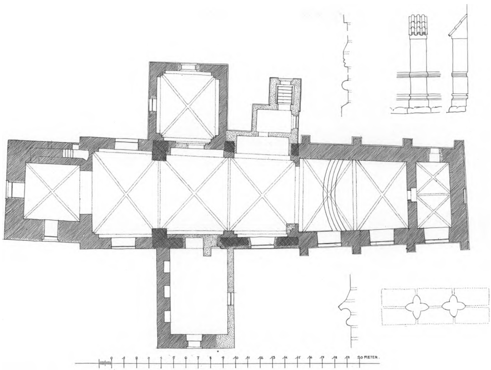
Fig. 6. Plan 1:300 med følgende detaljer fra koret: støttepille (1:150), profil af sokkel og bæltegesims, profil af gavlens gesims samt fordybninger herunder (1:30). Målt og tegnet af Charles Christensen 1921. Signaturforklaring s. 9. - Ground-plan with architectural details of the chancel: pier, mouldings of base, string-course and cornice of gable with recesses below it. Key on p. 9.
