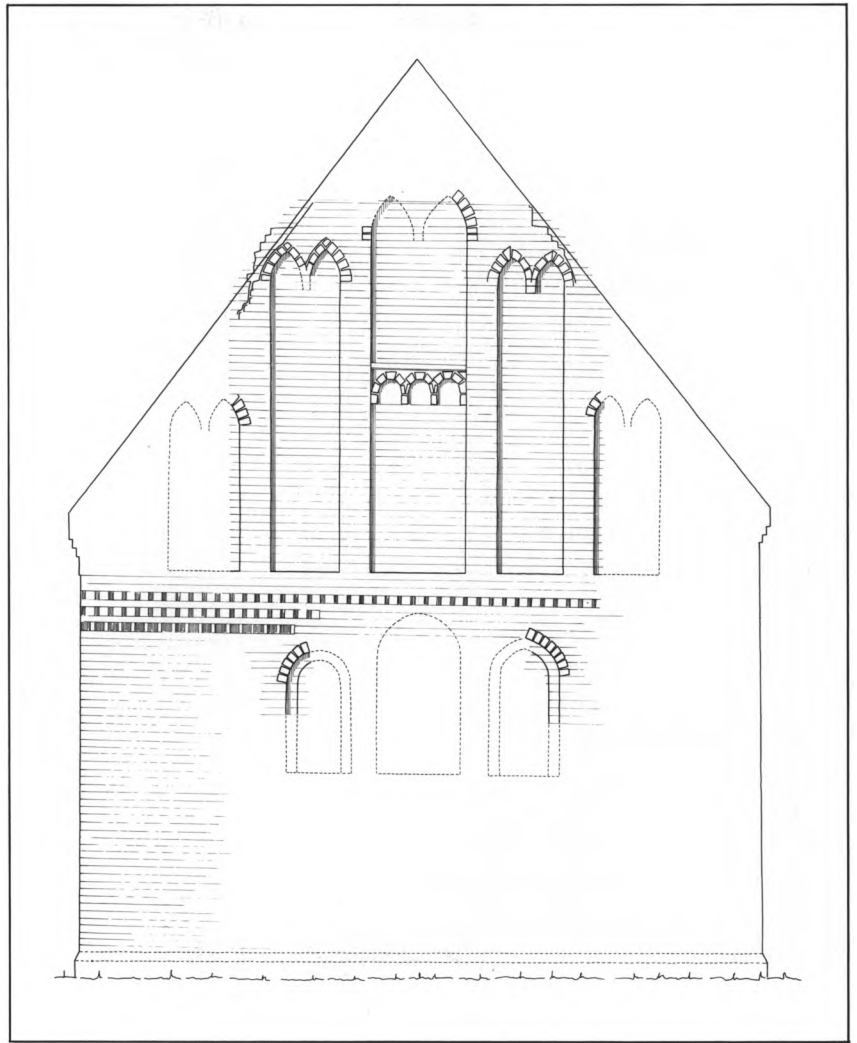
Fig. 10. Vestforlængelsens gavl med levn af blændingsdekoration, set fra de to mellemstokværk. Angivet er tillige levn af vinduer, som er synlige på gavlens inderside (s. 1448). 1:100. Målt ved HeJ 1985 og tegnet af Marianne Nielsen 1986. - Gable of the west extension with remains of recesses, seen from the two middle storeys of the tower. Traces of windows are visible on the inner face of the gable.
