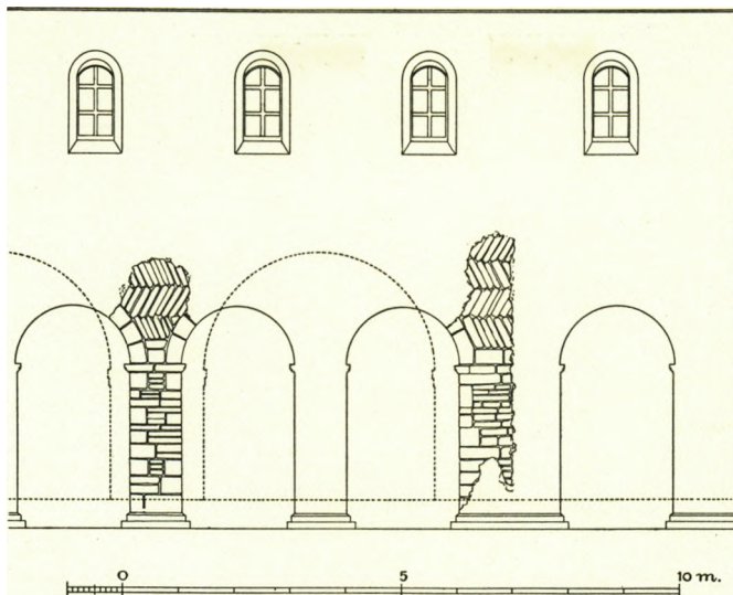
Fig. 8. Roskilde Vor Frue. Rekonstruktion af den vestligste Del af søndre Midtskibsvæg; den senere Arkadedeling og nuværende Gulvhøjde indpunkteret. 1:150. Tegnet af C. G. S. 1944 paa Grundlag af Korerup og Undersøgelser 1933—34 (S. 66).
