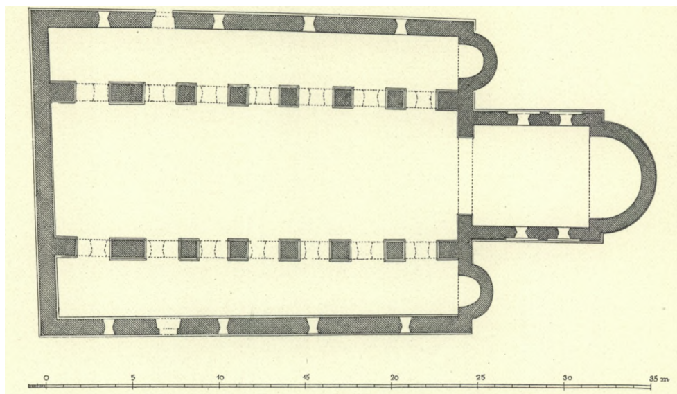
Fig. 7. Roskilde Vor Frue. Den oprindelige Bygning. Rekonstruktionsplan. 1:300. Maalt og tegnet af C. G. S. 1933—34.
