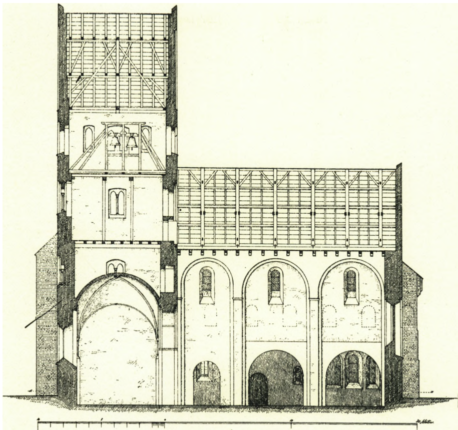
Fig. 9. Roskilde Vor Frue. Langsnit. 1:300. Efter Löffler: Sjællands Stiftslandsbykirker.
