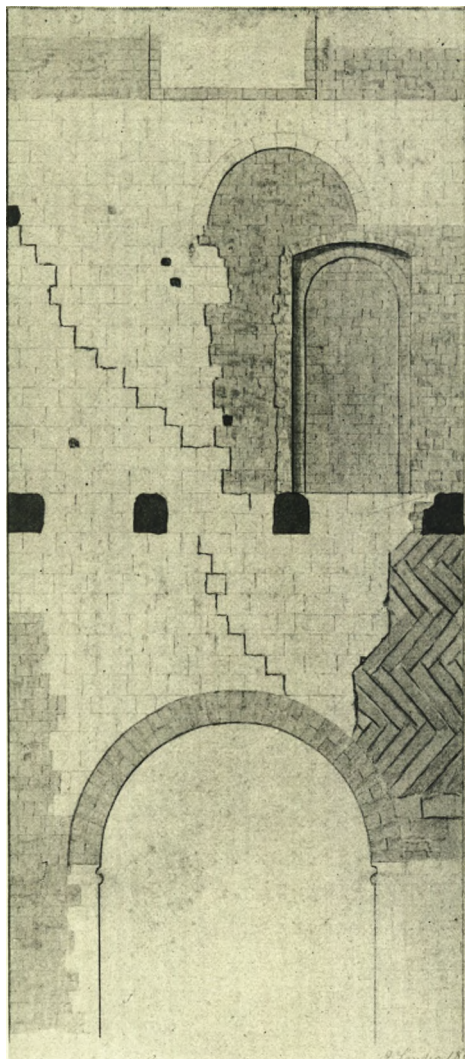
Fig. 11. Roskilde Vor Frue. Parti af Skibets nordre Sidemur. Farvelagt Tegning af I. Landtner 1865 (S. 66, 75).
