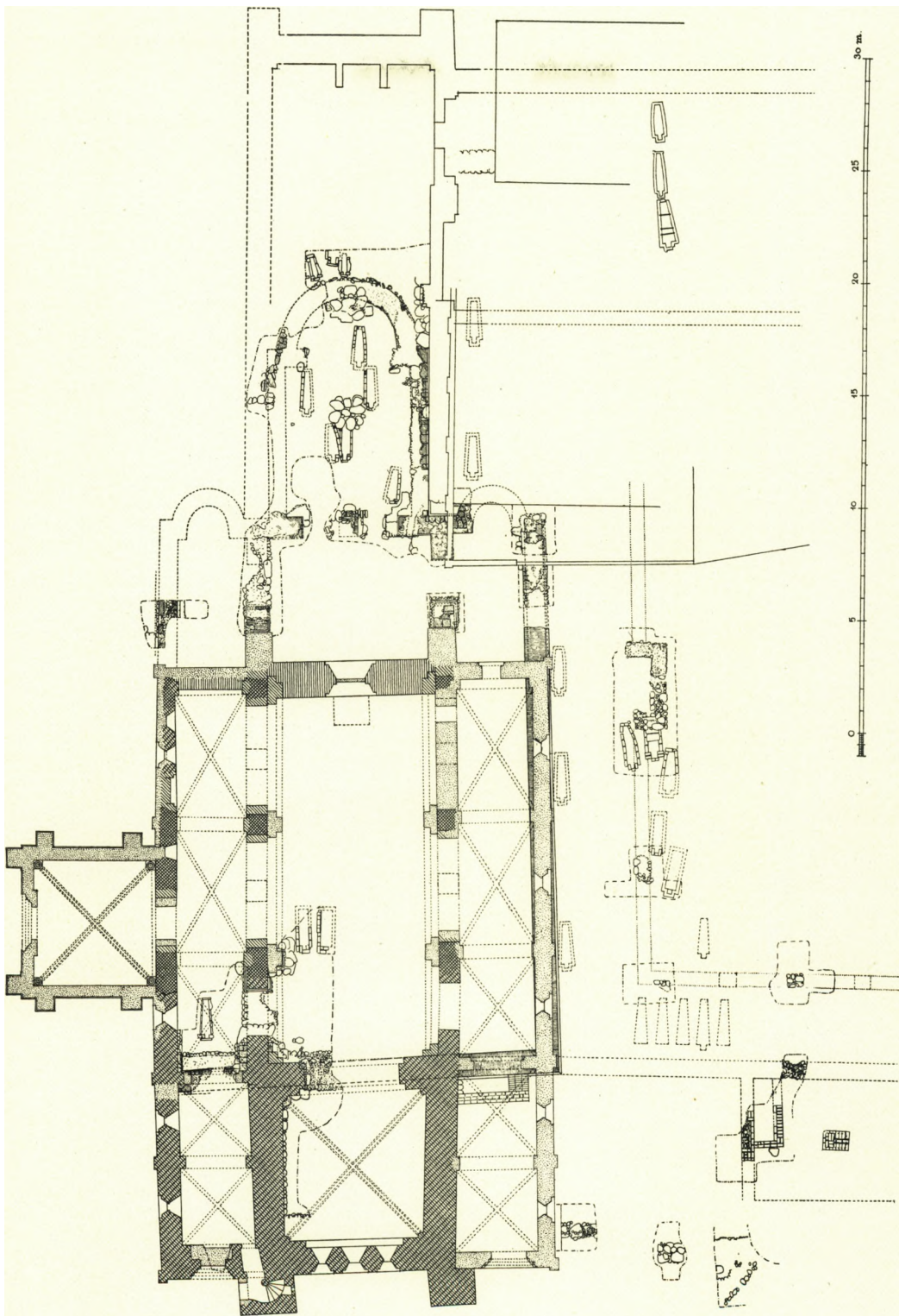
Fig. 2. Roskilde Vor Frue. Udgravningsplan. 1:300. Maalt af C. G. S. 1935.
