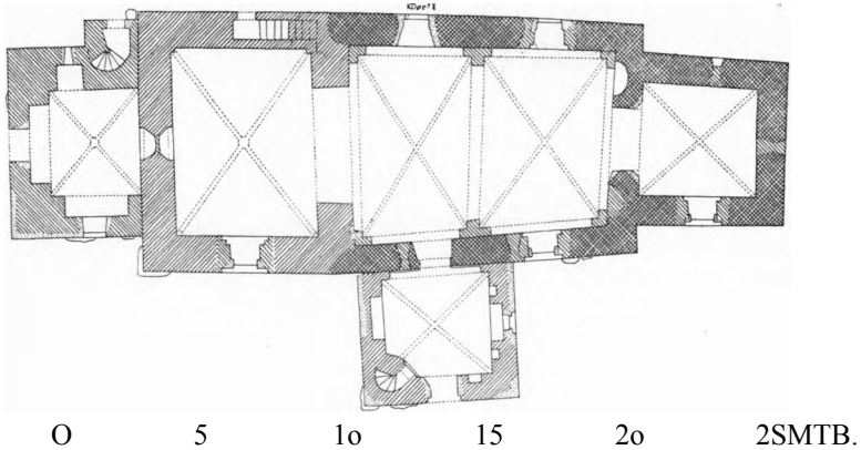
Fig. 2. Tune. Plan 1:300. Maalt af C. G. S. 1934.
