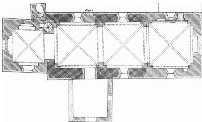
Fig. 2. Gadstrup. Plan 1:300. Maalt af A. Nystrøm 1929.
