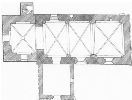
Fig. 2. Kimmerslev. Plan 1:300. Maalt af A. Nystrom 1929 (El. M. 1946).
