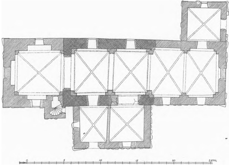
Fig. 2. Højelse. Plan 1:300. Maalt af A. Nystrom 1929.
