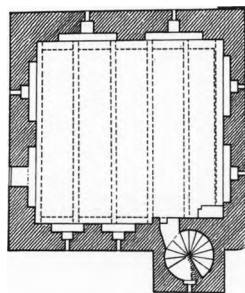
Fig. 3. Højelse. Plan af Taarnets Mellemstokværk 1:300. Maalt af Claudi-Hansen 1911.
