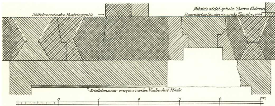
Fig. 6 a—b. Taarnby. Opstalt og Plan af den romanske Bygning's Nordmur, vestlige Del (bag Vaabenhus). 1:50. Maalt af El. M. 1944—45.
