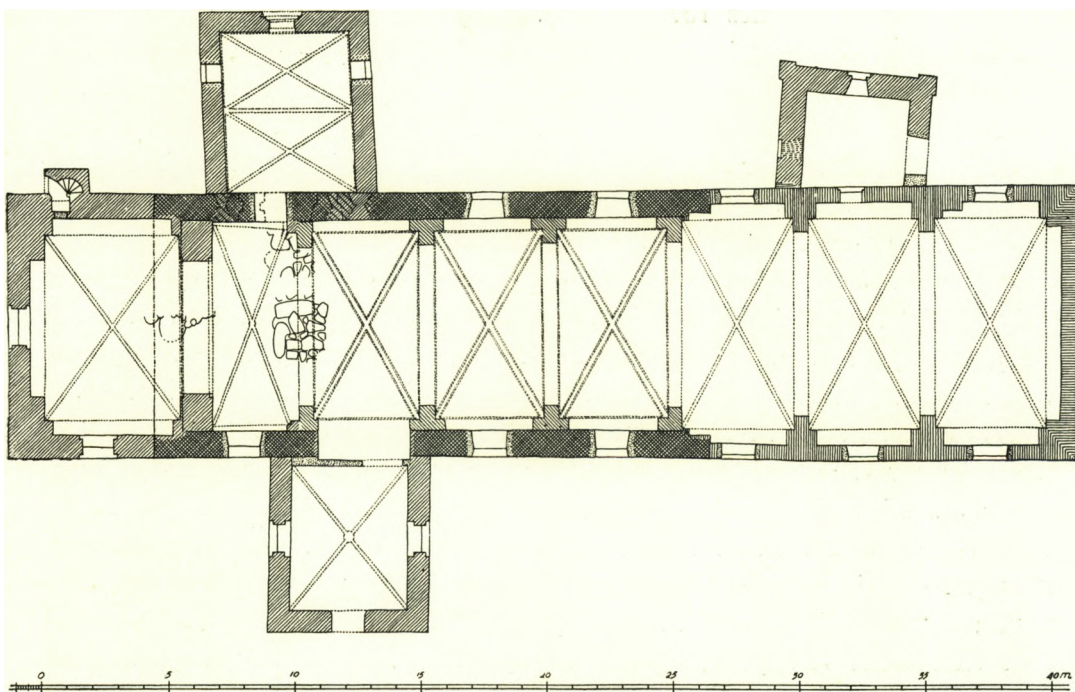
Fig. 2. Taarnby. Plan. 1:300. Maalt af El. M. 1942 (1944).
