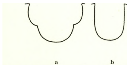
Fig. 2. Taarnby. Førmåsten og Dørprofil a — c. Ribbeprofiler. 1:10. a. Oprindeligt Skib (S. 284), b. Østforlængelse (S. 288), c. Søndre Tilbygning (S. 286), d. Profilgesims. 1:20. Søndre Tilbygning (S. 285), e. Dørprofil. 1:20 nordre Vaabenhus (S. 284). Maalt af El. M. 1944.
