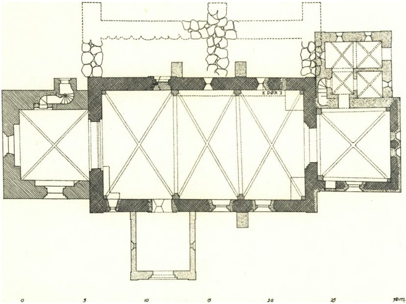
Fig. 2. Brønshøj. Plan. 1:300. Maalt af C. G. S. 1937, med indtegnede Fundamenter efter Opmaaling af Herholdt (El. M. 1945).
