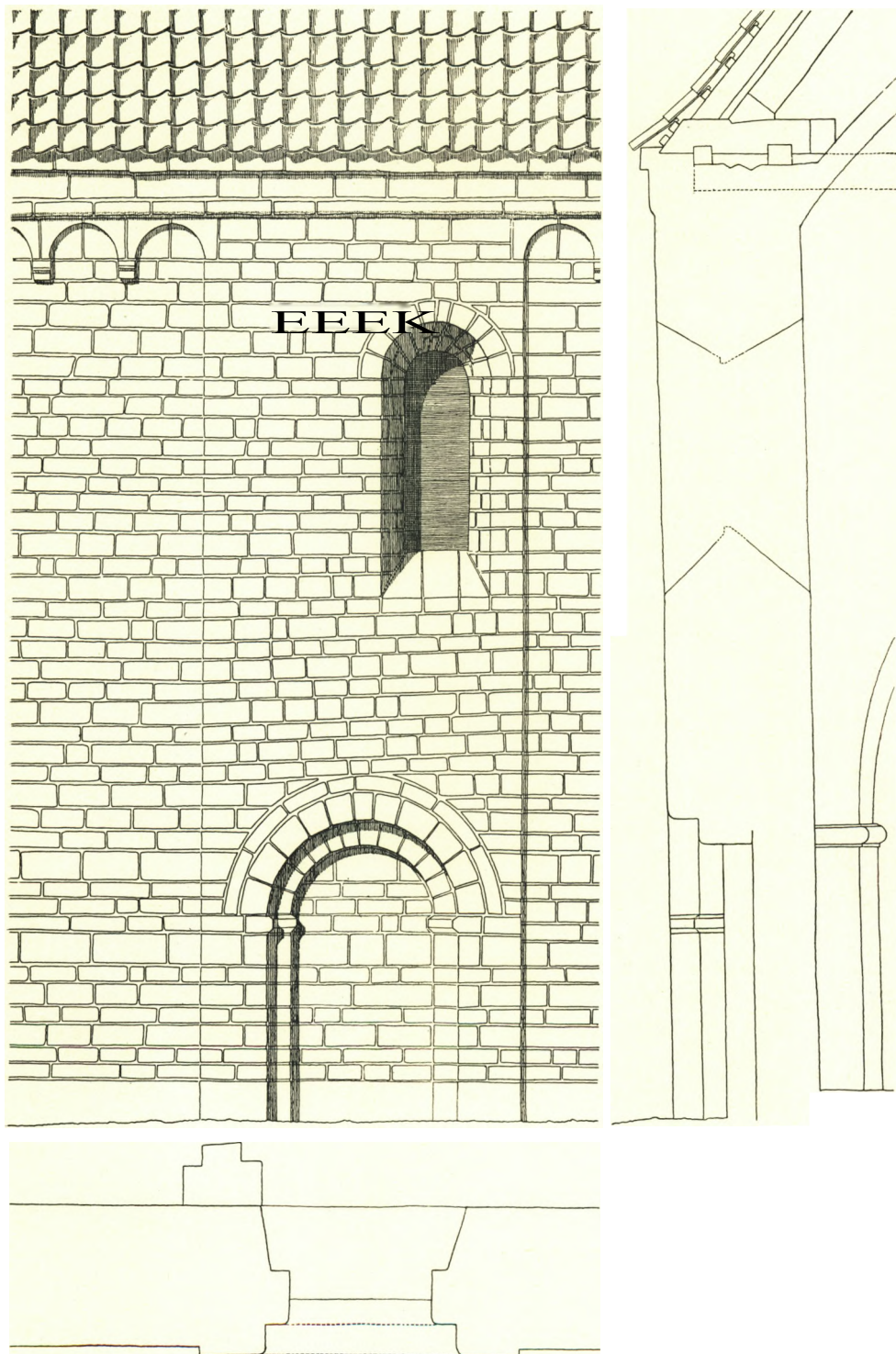
Fig. 5. Brønshøj. Detail af Skibets Nordmur. 1 : 50. Maalt af V. Hardie Fischer.
