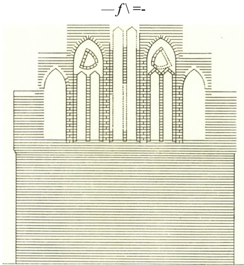
Fig. 3. Herlev. Oprindelig Vestgavl. Opmaaling og Rekonstruktion. 1: 150. Maalt af El. M. 1945 (S. 375).
