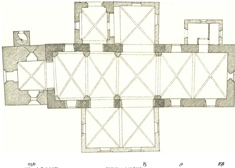
Fig. 2. Søllerød. Plan. 1:300. Maalt af Arne Nystrom 1937.
