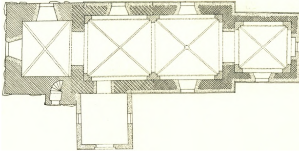
Fig. 2. Vallengsbæk. Plan. 1 : 300. Maalt af C. G. S. 1936. Vestpartiet er skraveret senromansk, men Dateringen er usikker.
