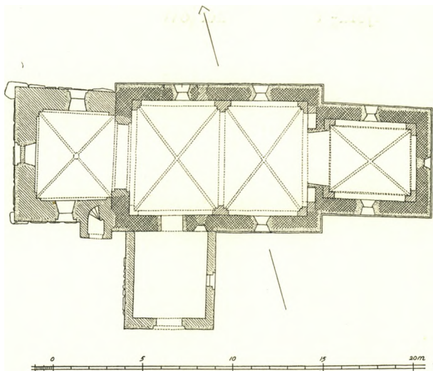
Fig. 2. Ishøj. Plan. 1:300. Maalt af El. M. 1943.
