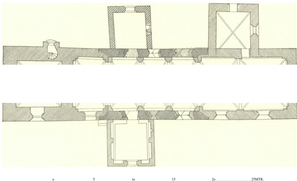
Fig. 2. Høje-Taastrup. Plan. 1:300. Maalt af C. G. S. 1934.
