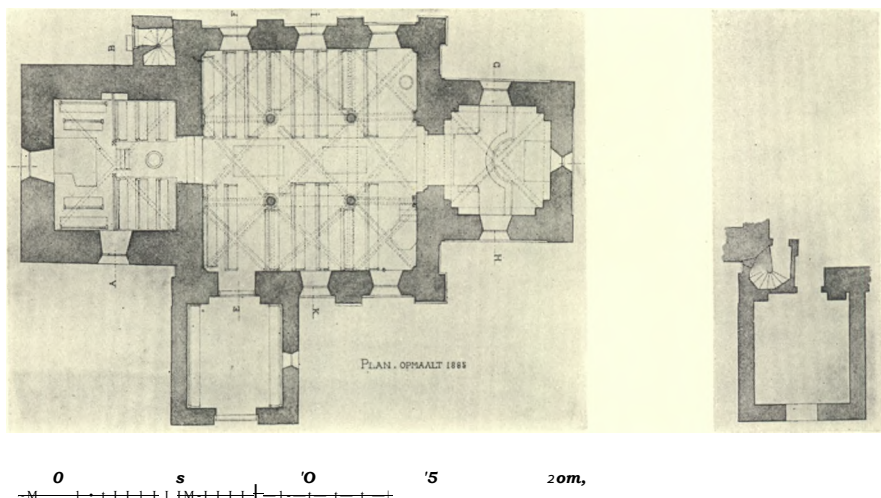
Fig. 2a-b. Ledøje. Planer 1:300. Før Restaureringen. 2 a. Underkirken. 2 b. Trappens Udmunding i Overkirken. Maalt af H. B. Storck 1885.
