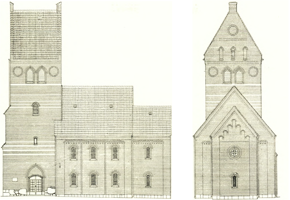
Fig. 12-13. Ledøje. Syd- og Østfaçade. 1:300. Nuværende Tilstand. Maalt af S. Albinus 1926.
