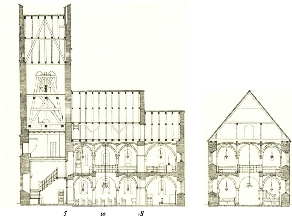
Fig. 6-7. Ledøje. Længdesnit og Tværsnit. 1:300. Nuværende Tilstand. Maalt 1926 af S. Albinus.
