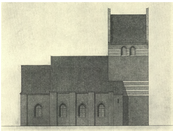
Fig. 8. Ledøje. Nordfaçade. 1:300. Maalt af Hoffmann 1862.
