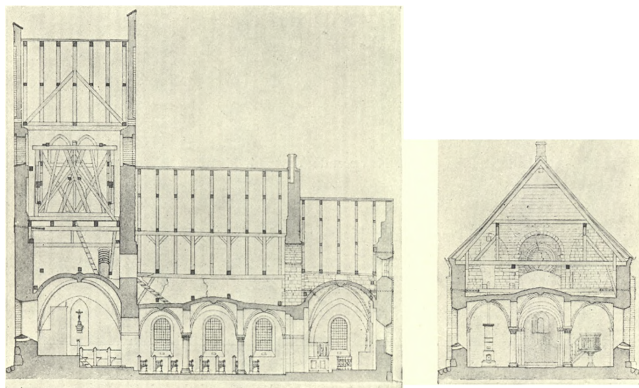
Fig. 4-5. Ledøje. Længdesnit og Tværsnit. 1:300. Før Restaureringen. Maalt af H. B. Storck 1885.
