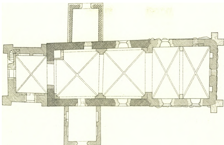
Fig. 2. Smørum. Plan. 1:300. Maalt af Paul Momme 1925 (El. M. 1946).
