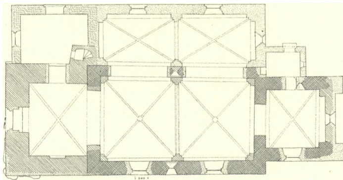
Fig. 2. Ballerup. Plan. 1:300. Maalt af Charles Christensen 1921 (El. M. 1945).
