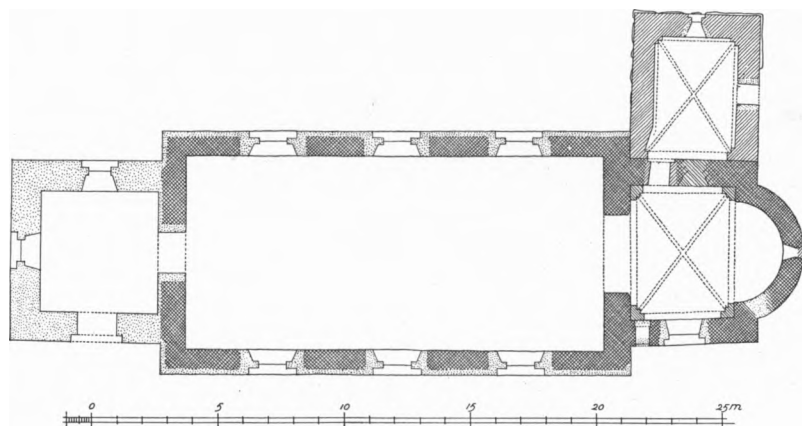
Fig. 2. Kirke-Hyllinge. Plan. 1:300. Maalt af El. M. 1946.
