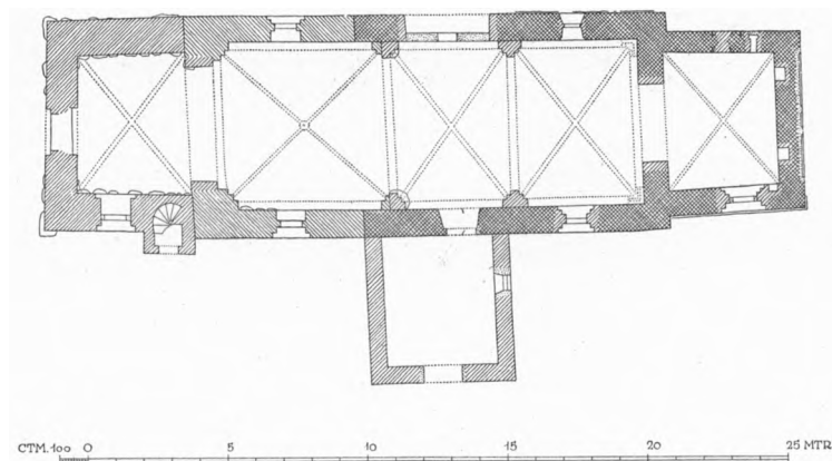
Fig. 2. Gershøj. Plan. 1:300. Maalt af C. G. S. 1932.
