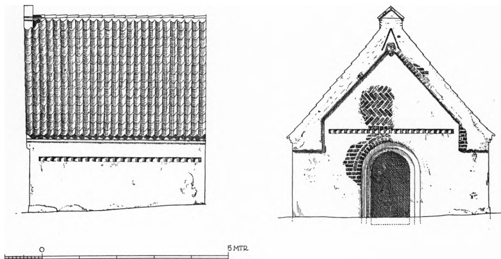
Fig. 6—7. Greve. Vaabenhus, Vestside og Gavl. 1:100. Maalt af C. G. S. 1930 (S. 961).
