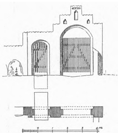
Fig. 3. Greve. Kirkegaardens Nordportal. 1:150. Maalt af Knud Barfoed 1915. Graven under \dagger Kirkerist i Laagen indtegnet af El. M. (S. 959).
